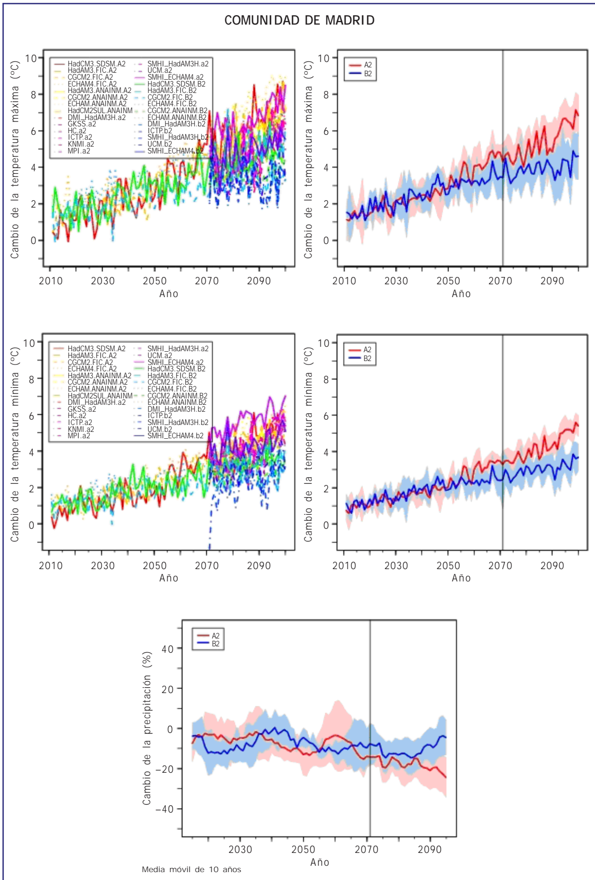
Figura B13. Igual que Figura B1, pero para la Comunidad de Madrid.
