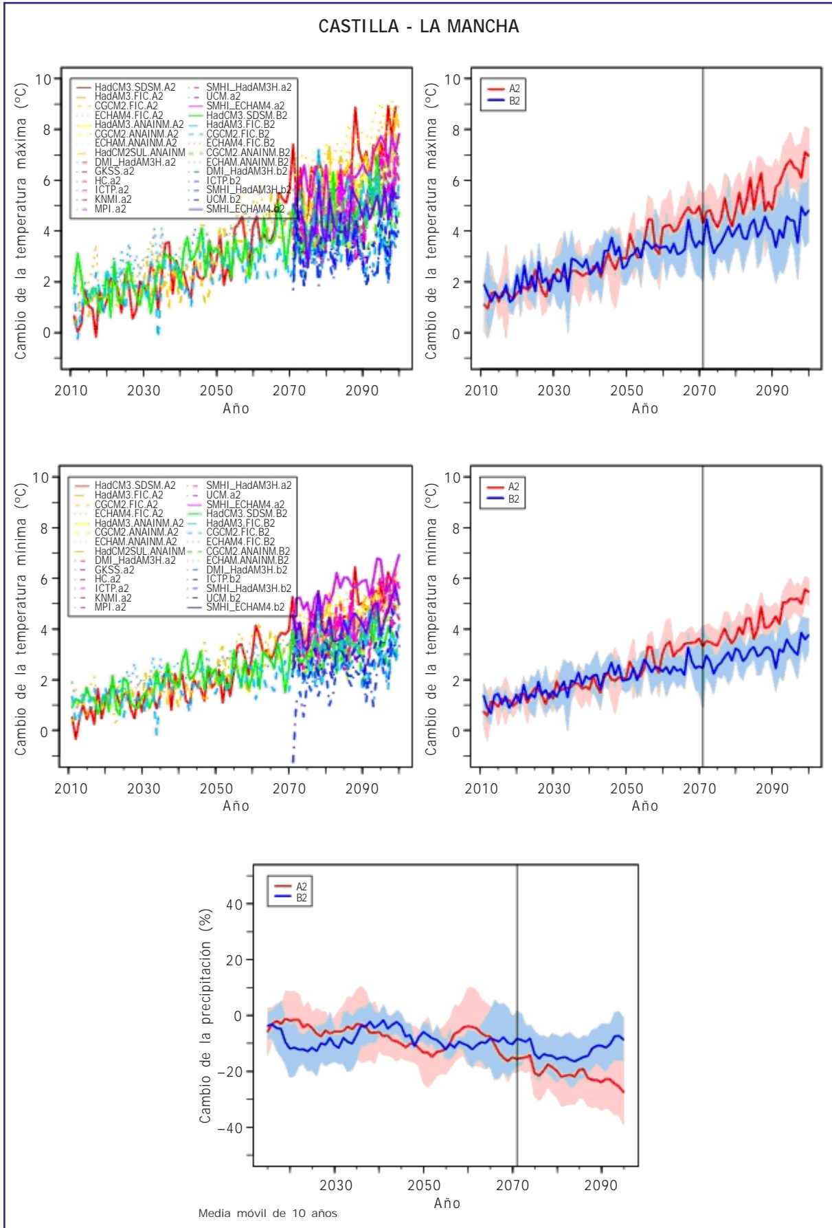
Figura B7. Igual que Figura B1, pero para Castilla - La Mancha.
