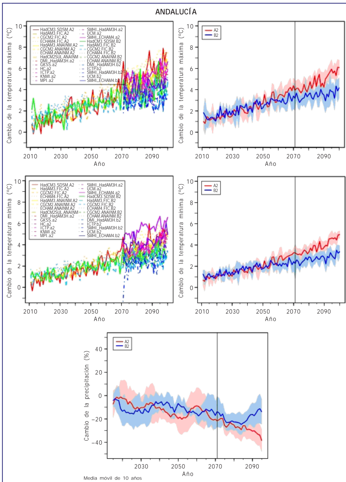
Figura B1. Evolución del cambio de Tmax (arriba izda.) y Tmin (centro izda.) anual media en Andalucía obtenido con diferentes modelos globales, técnicas de regionalización y escenarios de emisión respecto al valor promedio de referencia en el período 1961-1990. Evolución del valor medio (curva continua) y valor medio +/- desviación estándar (sombreado) para Tmax (arriba der.), Tmin (centro der.) y precipitación (abajo). (La curva correspondiente al valor medio de la precipitación representa la media móvil centrada para un período de 10 años).
