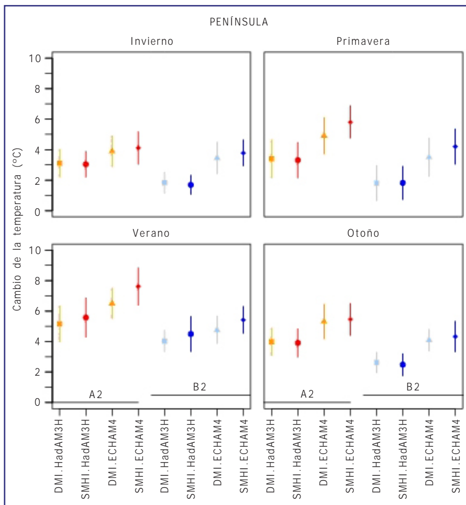
Figura 3.2. Valor medio de la diferencia de temperatura del período 2071-2100 respecto al período 1961-1990 para la España peninsular en invierno, primavera, verano y otoño. Este valor se ha estimado a partir de dos modelos regionales (DMI y SMHI), dos modelos globales (HadAM3H y ECHAM4/OPYC) y dos escenarios de emisión (A2 y B2). Cada barra indica la separación en \pm 1 desviación estándar respecto de la media.
