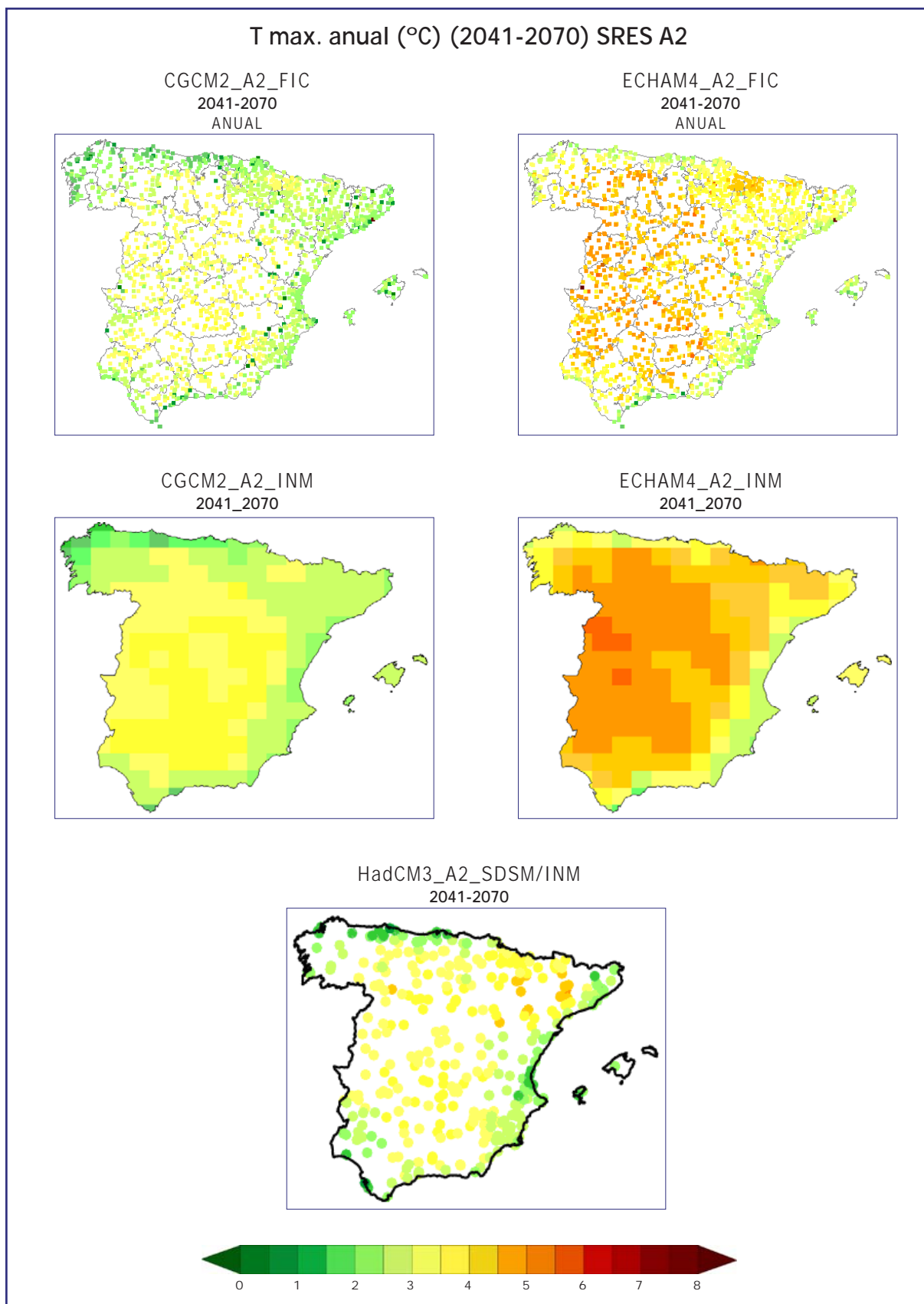
Figura 6.2. Comparación del cambio de temperatura máxima media anual para el período 2041-2070 respecto al período de control (1961-90) proporcionado por las proyecciones regionalizadas utilizando diferentes modelos globales (CGCM2 (izda.), ECHAM4-OPYC (der.), HadCM3 (centro abajo) y diferentes técnicas de regionalización estadísticas (Anal_FIC (arriba), Anal_INM (centro), SDSM (abajo)). El escenario de emisión SRES común a todos los modelos es el A2.
