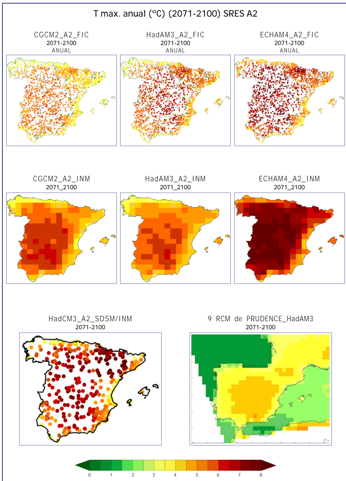
Figura 6.3. Comparación del cambio de temperatura máxima media anual para el período 2071-2100 respecto al período de control (1961-90) proporcionado por las proyecciones regionalizadas utilizando diferentes modelos globales (CGCM2 (izda.), ECHAM4-OPYC (der.), HadAM3 (centro), HadCM3 (abajo izda.)) y diferentes técnicas de regionalización estadísticas (Anal_FIC (arriba), Anal_INM (centro), SDSM (abajo izda.)) y dinámicas (promedio de los 9 RCM de PRUDENCE (abajo der.)). El escenario de emisión SRES común a todos los modelos es el A2.
