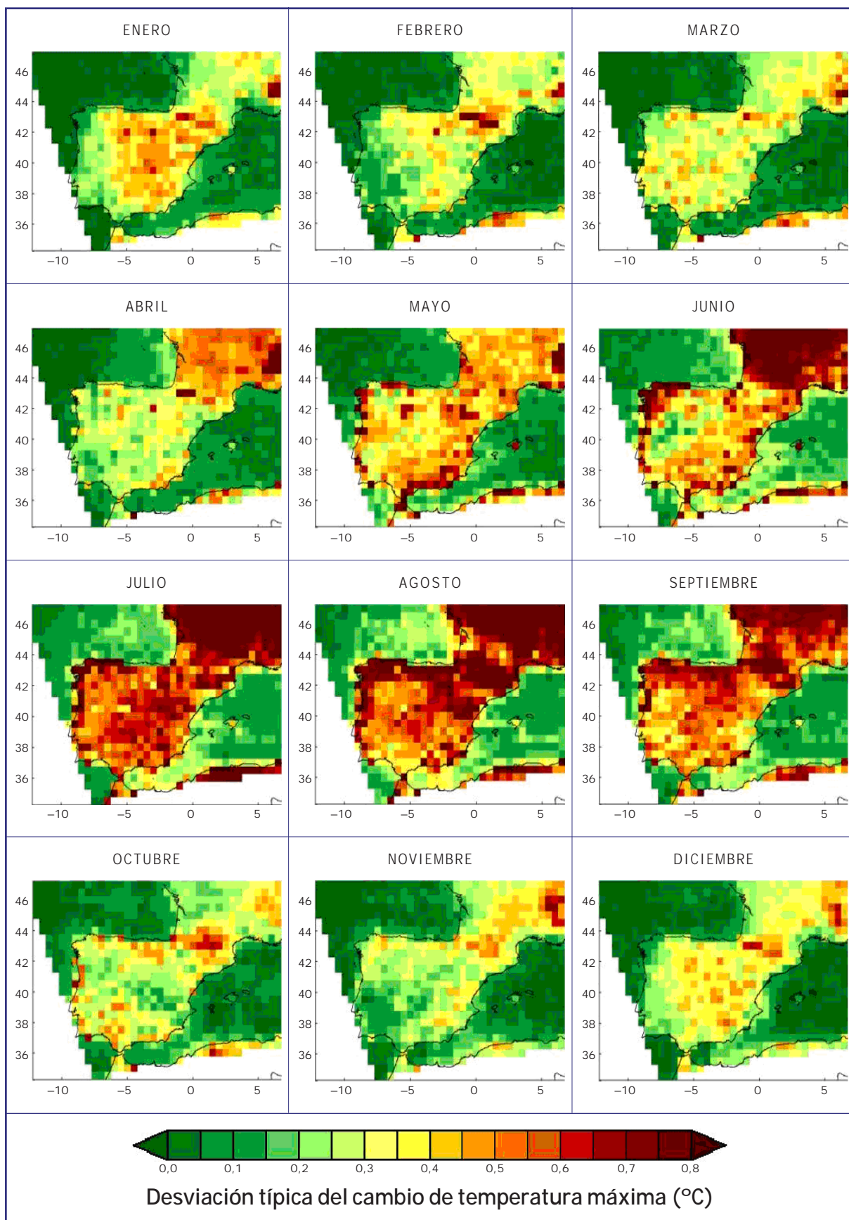
Figura 6.10. Distribución mensual de la desviación típica del cambio proyectado en la temperatura máxima para los diez modelos regionales de PRUDENCE en el período 2071-2100 respecto al clima actual (1961-1990) y para el escenario de emisión SRES A2.
