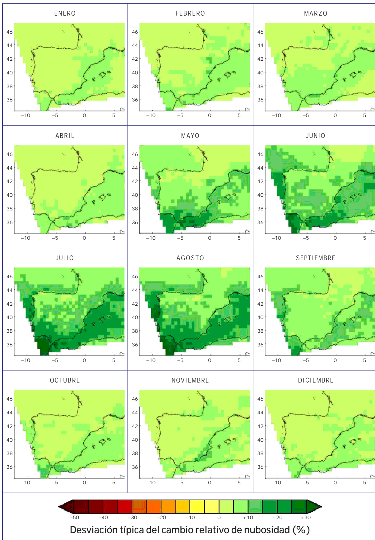
Figura 6.28. Distribución mensual de la desviación típica del cambio proyectado en la nubosidad (%) para los diez modelos regionales de PRUDENCE en el 2071-2100 respecto al clima actual (1961-1990) y para el escenario de emisión SRES A2.
