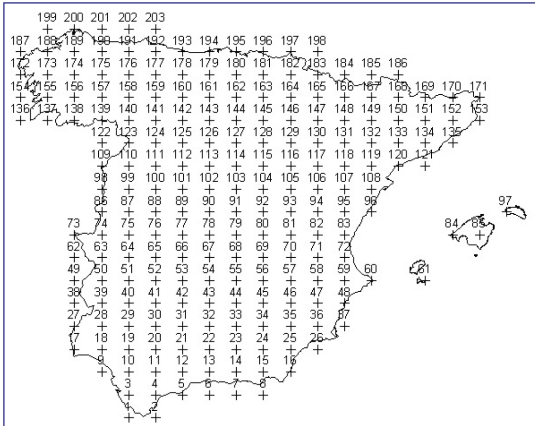
Figura 5.5. Rejilla de cálculo utilizada por el método de análogos INM.
