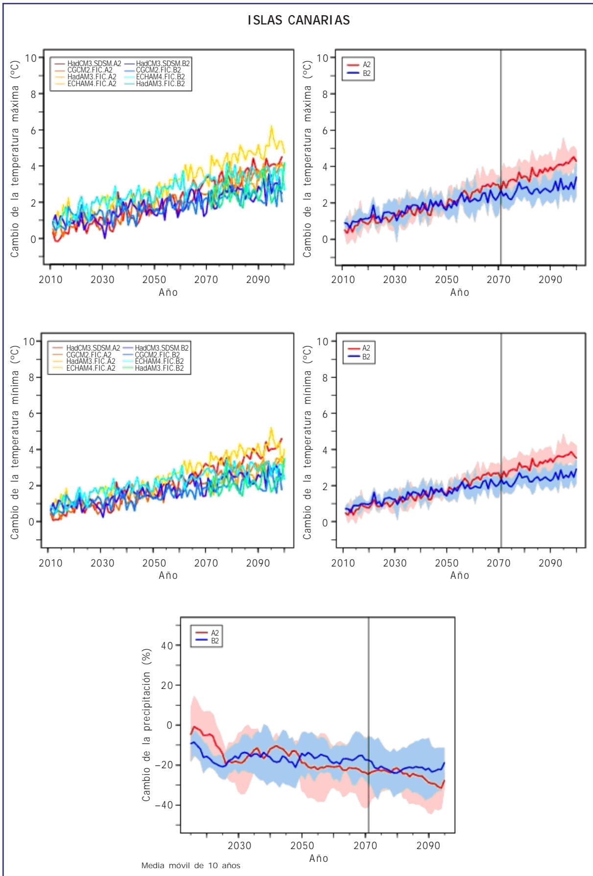
Figura B5. Igual que Figura B1, pero para las Islas Canarias.
