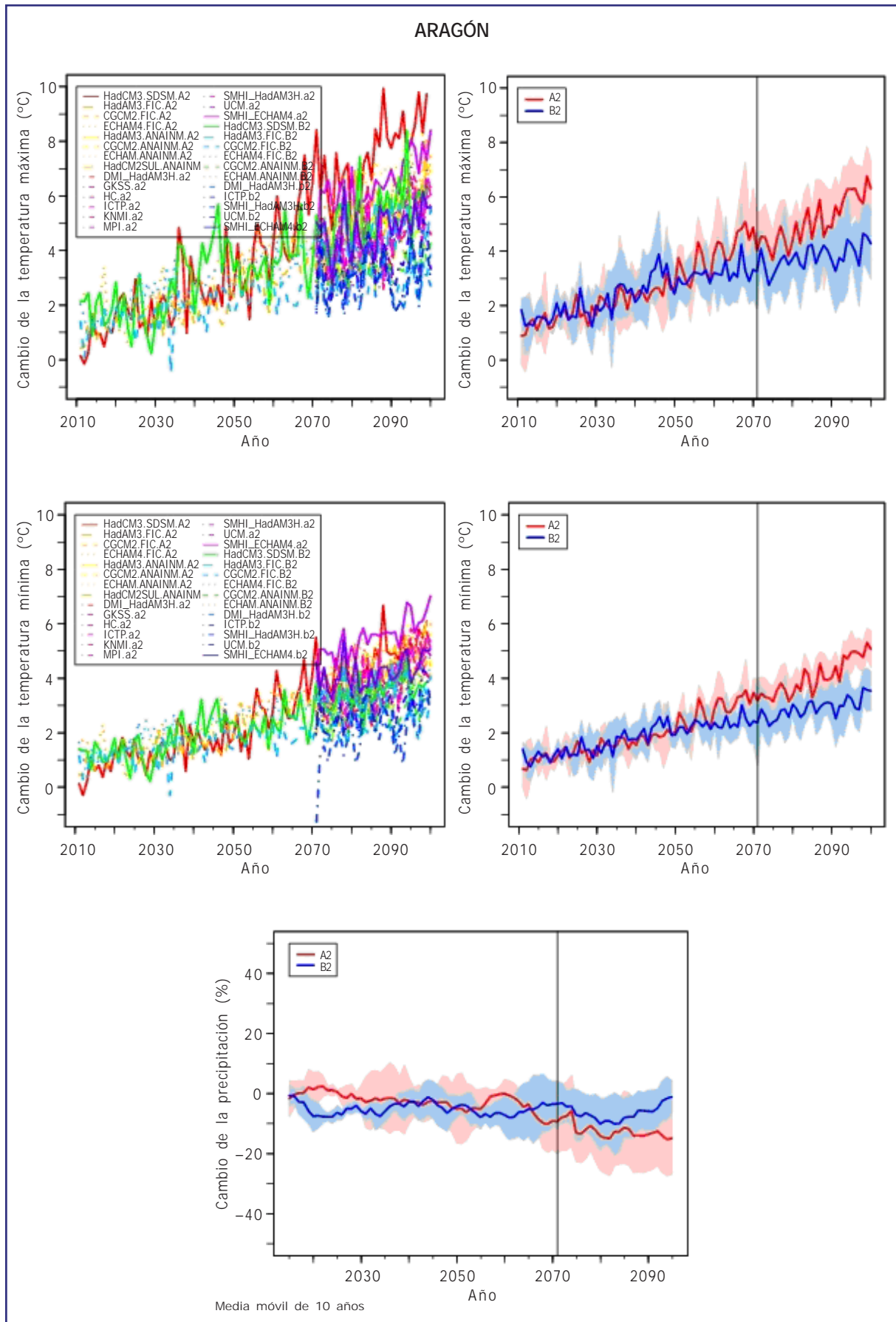
Figura B2. Igual que Figura B1, pero para Aragón.
