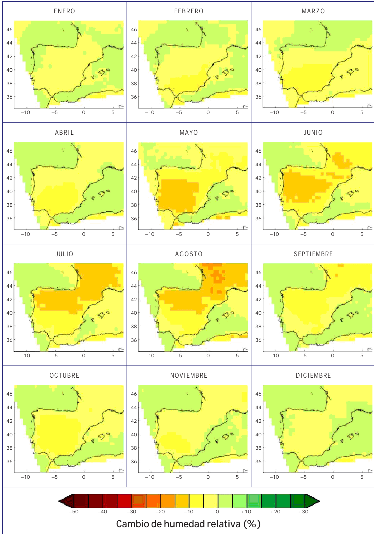
Figura 6.26. Cambio medio mensual de humedad relativa (%) proyectado para el período 2071-2100 respecto al clima actual (1961-1990) por el modelo global HadAM3H y regionalizado con el promedio de los RCM de PRUDENCE para el escenario de emisión A2.
