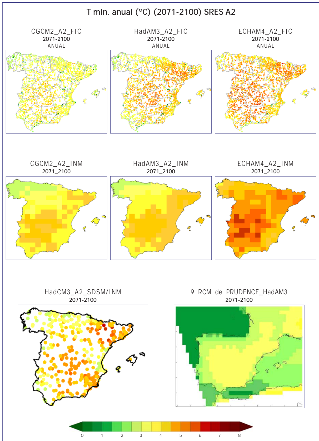
Figura 6.15. Comparación del cambio de temperatura mínima media anual para el período 2071-2100 respecto al período de control (1961-90) proporcionado por las proyecciones regionalizadas utilizando diferentes modelos globales (CGCM2 (izda.), ECHAM4-OPYC (der.), HadAM3 (centro), HadCM3 (abajo izda.)) y diferentes técnicas de regionalización estadísticas (Anal_FIC (arriba), Anal_INM (centro), SDSM (abajo izda.)) y dinámicas (promedio de los 9 RCM de PRUDENCE (abajo der.)). El escenario de emisión SRES común a todos los modelos es el A2.
