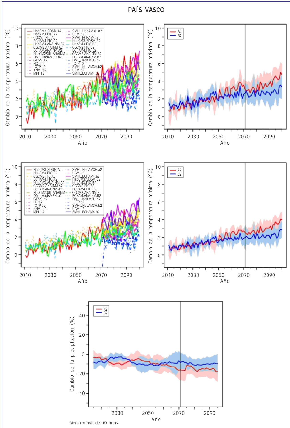
Figura B16. Igual que Figura B1, pero para el País Vasco.
