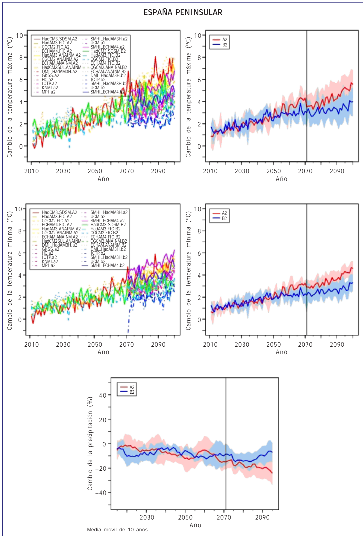
Figura B18. Igual que Figura B1, pero para España peninsular.
