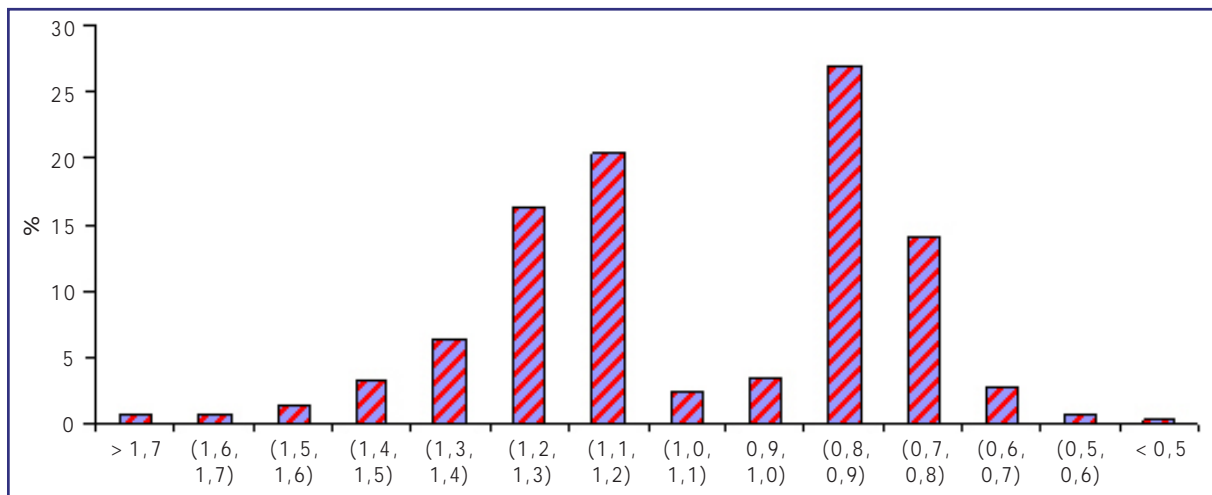
Figura 2.4. Histograma de la razón correctora para el test SNHT para las estaciones con inhomogeneidad al 5%.
