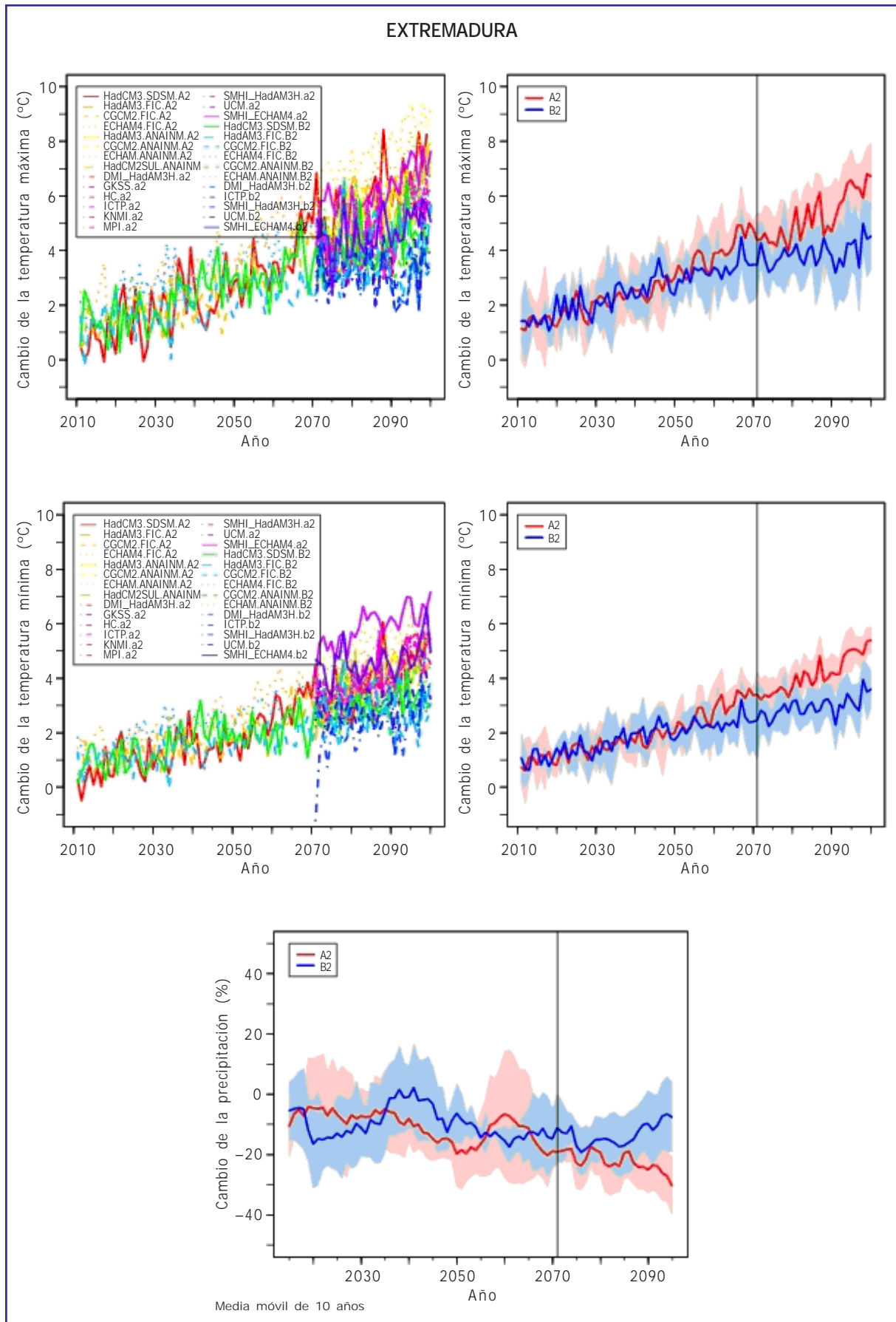
Figura B10. Igual que Figura B1, pero para Extremadura.
