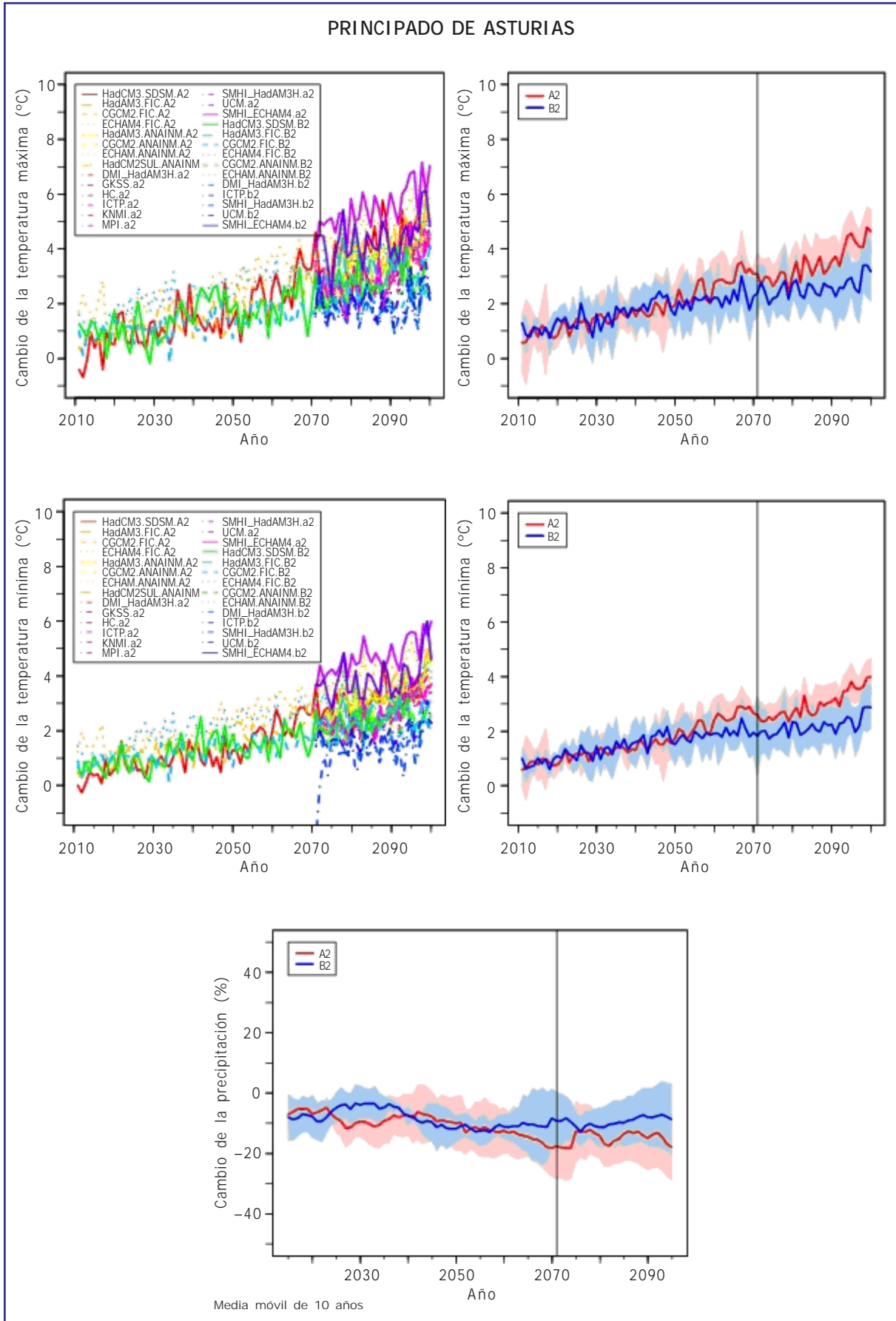
Figura B3. Igual que Figura B1, pero para el Principado de Asturias.
