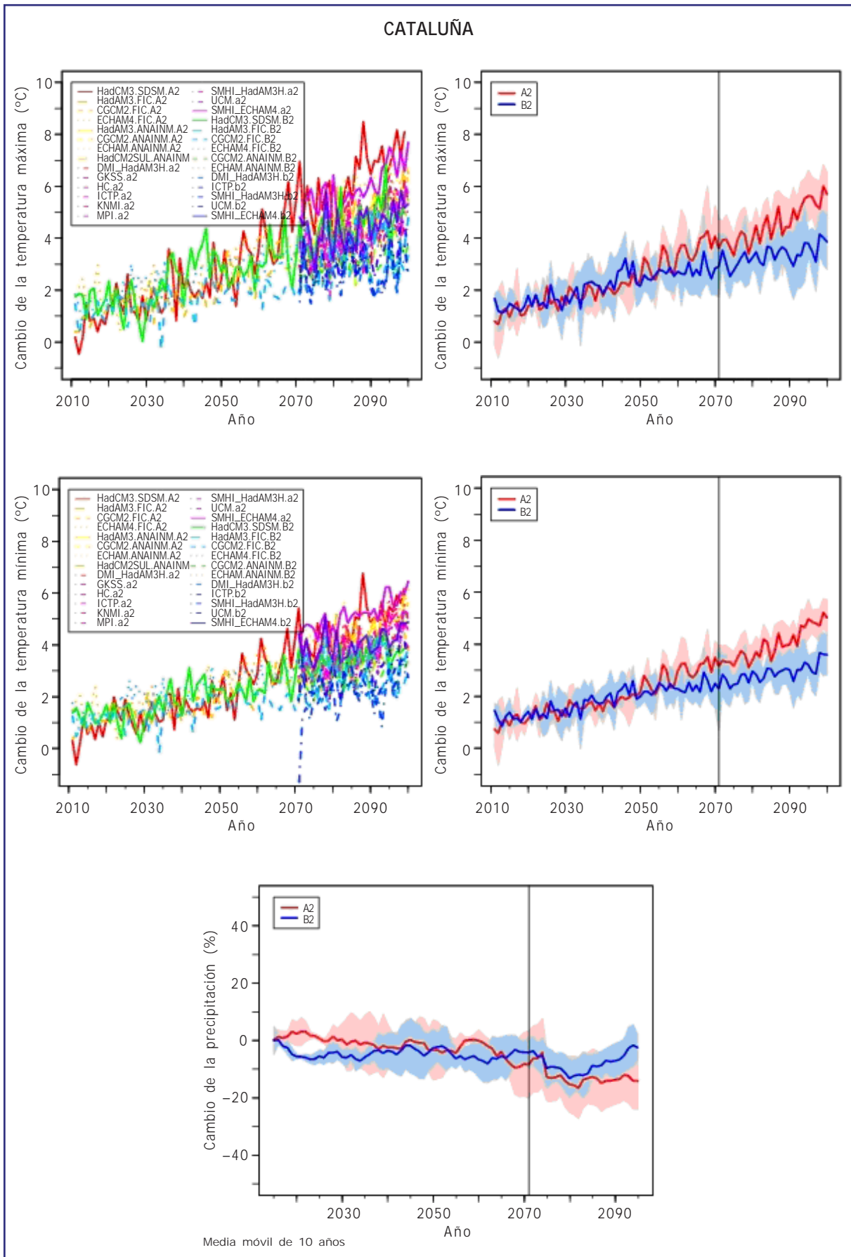
Figura B9. Igual que Figura B1, pero para Cataluña.
