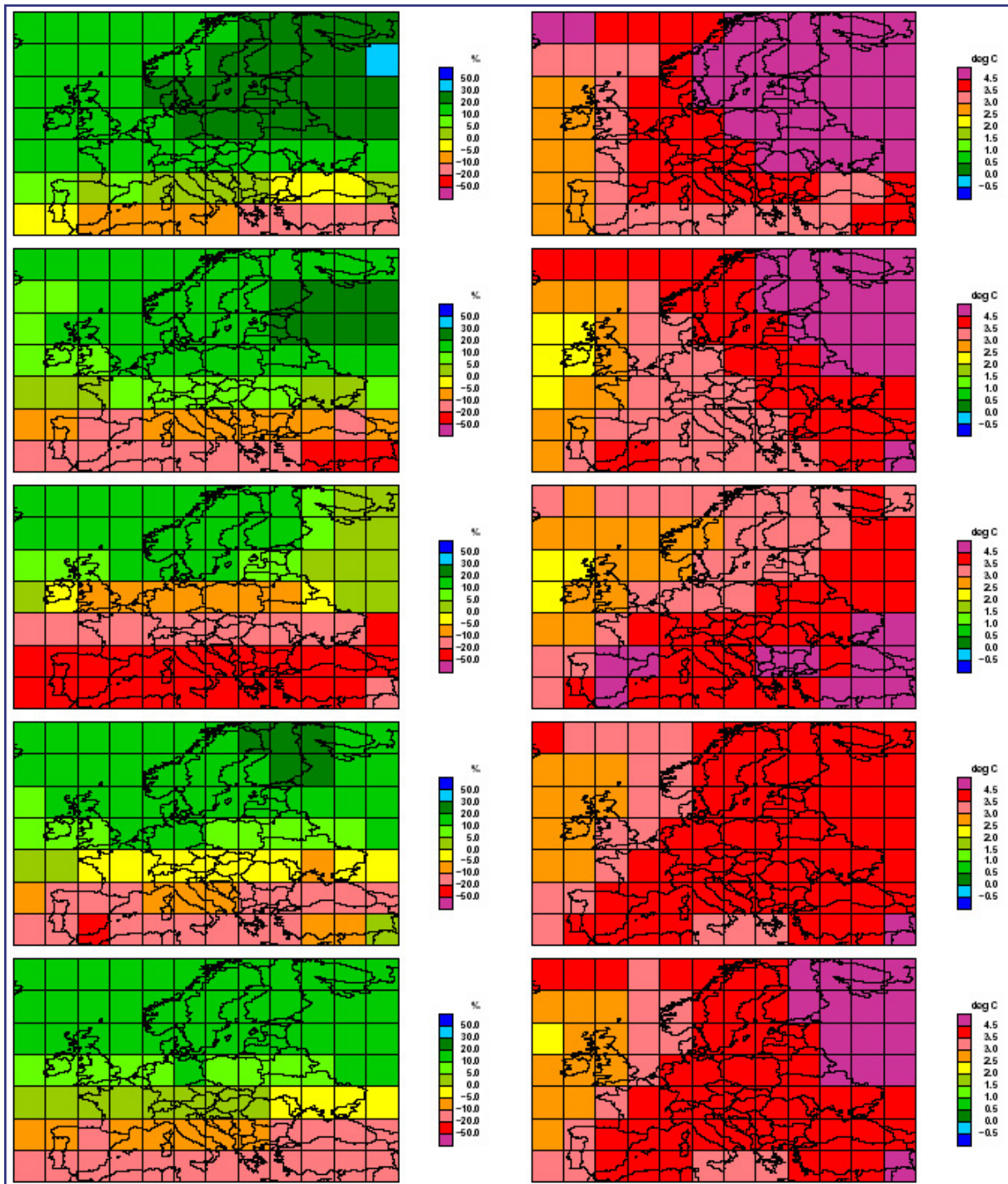
Figura 4.5. Cambio de precipitación (izquierda) y temperatura media (derecha) bajo el escenario de emisión SRES A2 para el período (2086-2015) con respecto al período de referencia (1961-1990) basado en el promedio de 16 AOCGM para invierno (fila 1.ª), primavera (fila 2.ª), verano (fila 3.ª), otoño (fila 4.ª) y para el promedio anual (fila 5.ª). Producido con MAGICC-SCENGEN (version 2.4) con la opción de sensibilidad climática media y los parámetros de MAGICC por defecto.
