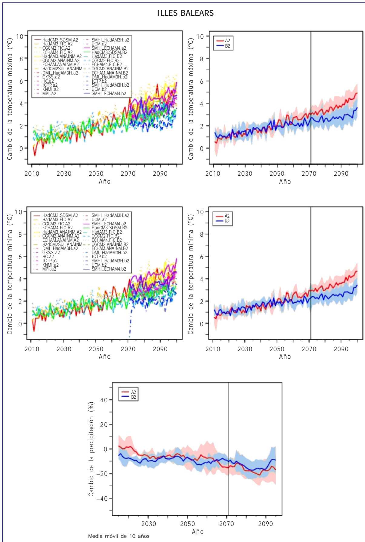
Figura B4. Igual que Figura B1, pero para las Illes Balears.
