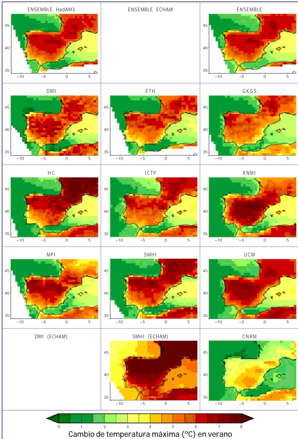
Figura 6.9. Igual que Figura 6.8, pero para verano (junio, julio, agosto).
