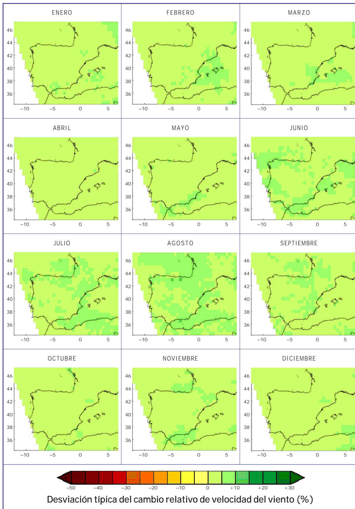
Figura 6.32. Distribución mensual de la desviación típica del cambio proyectado en la velocidad del viento (%) para los diez modelos regionales de PRUDENCE en el periodo 2071-2100 respecto al clima actual (1961-1990) y para el escenario de emisión SRES A2.
