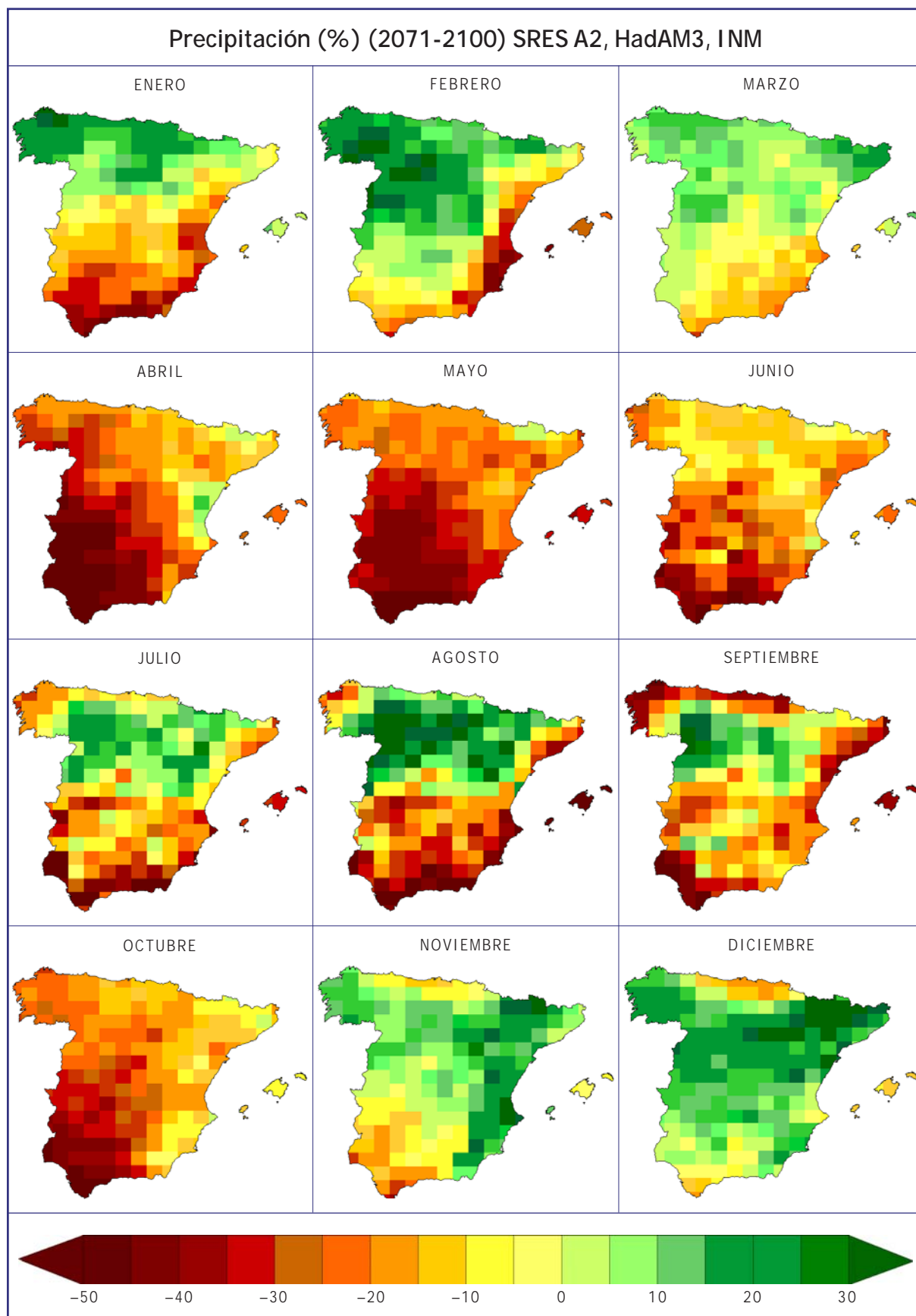
Figura 6.22. Cambio medio mensual de precipitación (%) proyectado para el periodo 2071-2100 respecto al clima actual (1961-1990) por el modelo global HadAM3 y regionalizado con el método de análogos (INM) para el escenario de emisión A2.
