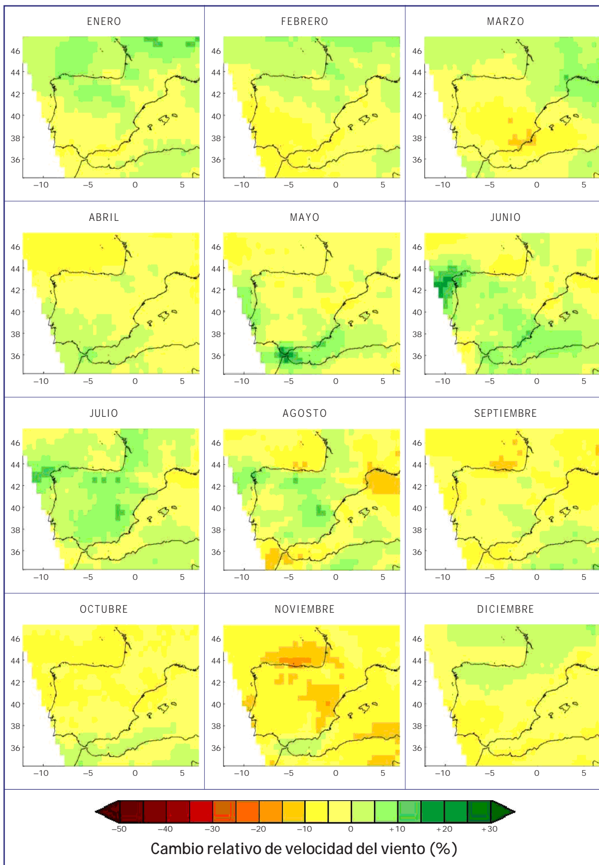
Figura 6.31. Cambio medio mensual de velocidad (%) proyectado para el período 2071-2100 respecto al clima actual (1961-1990) por el modelo global HadAM3H y regionalizado con el promedio de los RCM de PRUDENCE para el escenario de emisión A2.
