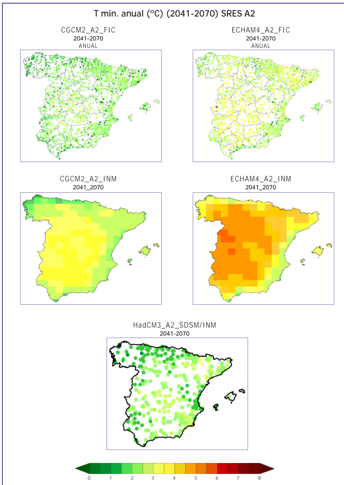
Figura 6.14. Comparación del cambio de temperatura mínima media anual para el período 2041-2070 respecto al período de control (1961-90) proporcionado por las proyecciones regionalizadas utilizando diferentes modelos globales (CGCM2 (izda.), ECHAM4-OPYC (der.), HadCM3 (centro abajo) y diferentes técnicas de regionalización estadísticas (Anal_FIC (arriba), Anal_INM (centro), SDSM (abajo)). El escenario de emisión SRES común a todos los modelos es el A2.
