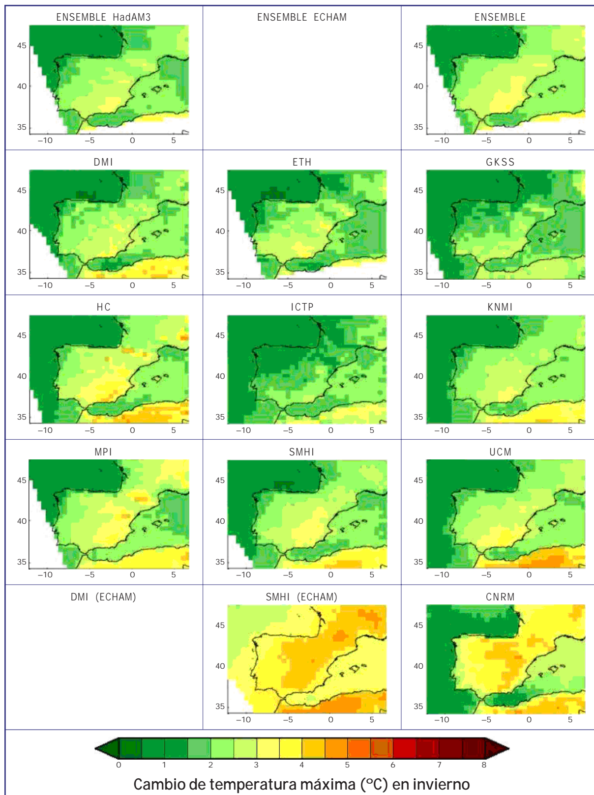
Figura 6.8. Distribución promedio estacional para invierno (diciembre, enero y febrero) de los cambios de temperatura máxima, respecto al clima actual (1961-1990), para 2071-2100 en el escenario A2, proyectado por: 1) cada uno de los modelos regionales de PRUDENCE anidados en los modelos globales HadAM3 ó ECHAM4, 2) por el promedio de todos los modelos regionales de PRUDENCE anidados en el HadAM3, 3) por el promedio de los modelos regionales de PRUDENCE anidados en el ECHAM4 y 4) por el promedio de todas las simulaciones con los modelos regionales. (Cuando no se indica lo contrario las simulaciones toman condiciones de contorno de HadAM3). Los datos de temperatura máxima para el modelo DMI anidado en ECHAM4 no están disponibles (Tabla A3).
