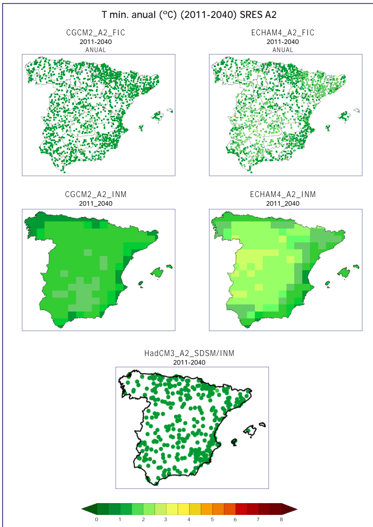
Figura 6.13. Comparación del cambio de temperatura mínima media anual para el período 2011-2040 respecto al período de control (1961-90) proporcionado por las proyecciones regionalizadas utilizando diferentes modelos globales (CGCM2 (izda.), ECHAM4-OPYC (der.), HadCM3 (centro abajo) y diferentes técnicas de regionalización estadísticas (Anal_FIC (arriba), Anal_INM (centro), SDSM (abajo)). El escenario de emisión SRES común a todos los modelos es el A2.
