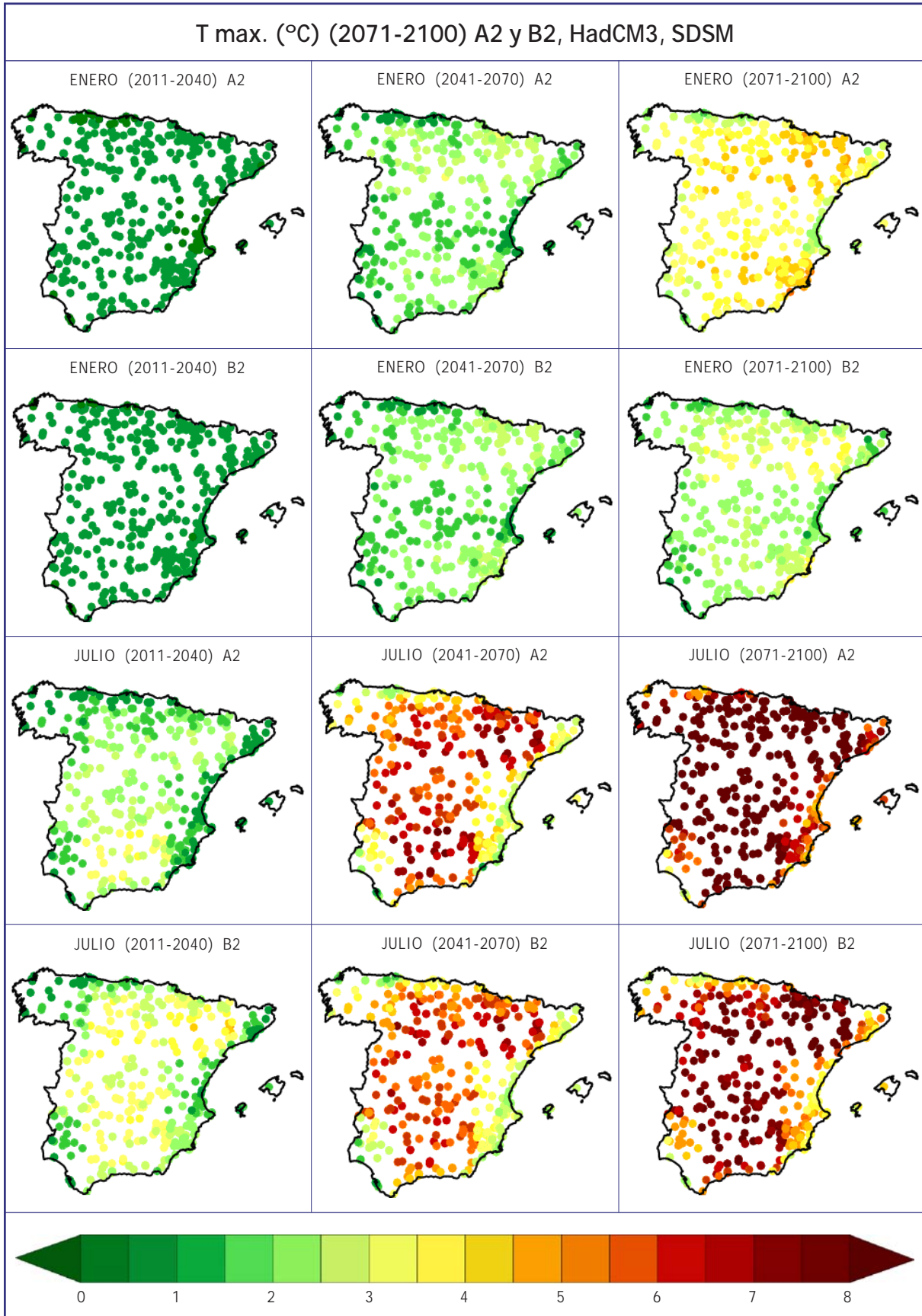
Figura 6.11. Cambio medio para enero (2 filas superiores) y julio (2 filas inferiores) de temperatura máxima proyectada por el modelo global HadCM3 para los períodos 2011-2040 (izda.), 2041-2070 (centro) y 2071-2100 (der.) respecto al clima actual (1961-1990) y regionalizado con el método de regresión (SDSM) para los escenarios de emisión SRES A2 y B2.
