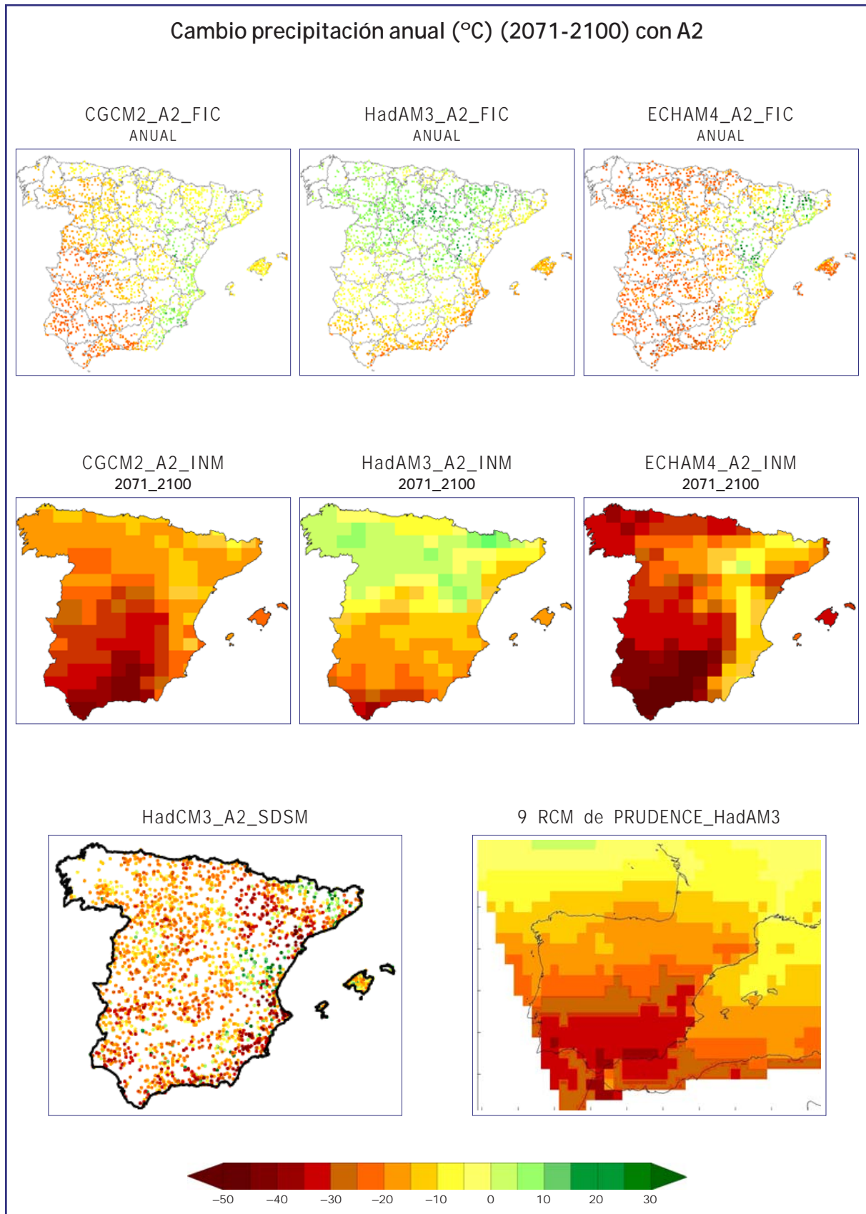
Figura 6.19. Comparación del cambio de precipitación anual para el período 2071-2100 respecto al período de control (1961-90) proporcionado por proyecciones regionalizadas utilizando diferentes modelos globales (HadCM3, HadAM3H, CGCM2, ECHAM4-OPYC) y diferentes técnicas de regionalización estadísticas (Anal_FIC, Anal_INM, SDSM) y dinámicas (promedio de los 9 RCM de PRUDENCE). El escenario de emisión SRES común a todos los modelos es el A2.
