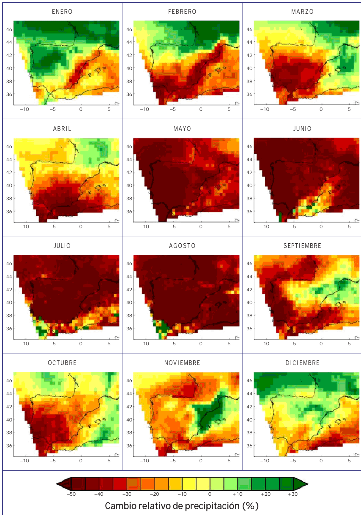
Figura 6.23. Cambio medio mensual de precipitación (%) proyectado para el periodo 2071-2100 respecto al clima actual (1961-1990) por el modelo global HadAM3H y regionalizado con el promedio de los RCM de PRUDENCE para el escenario de emisión A2.
