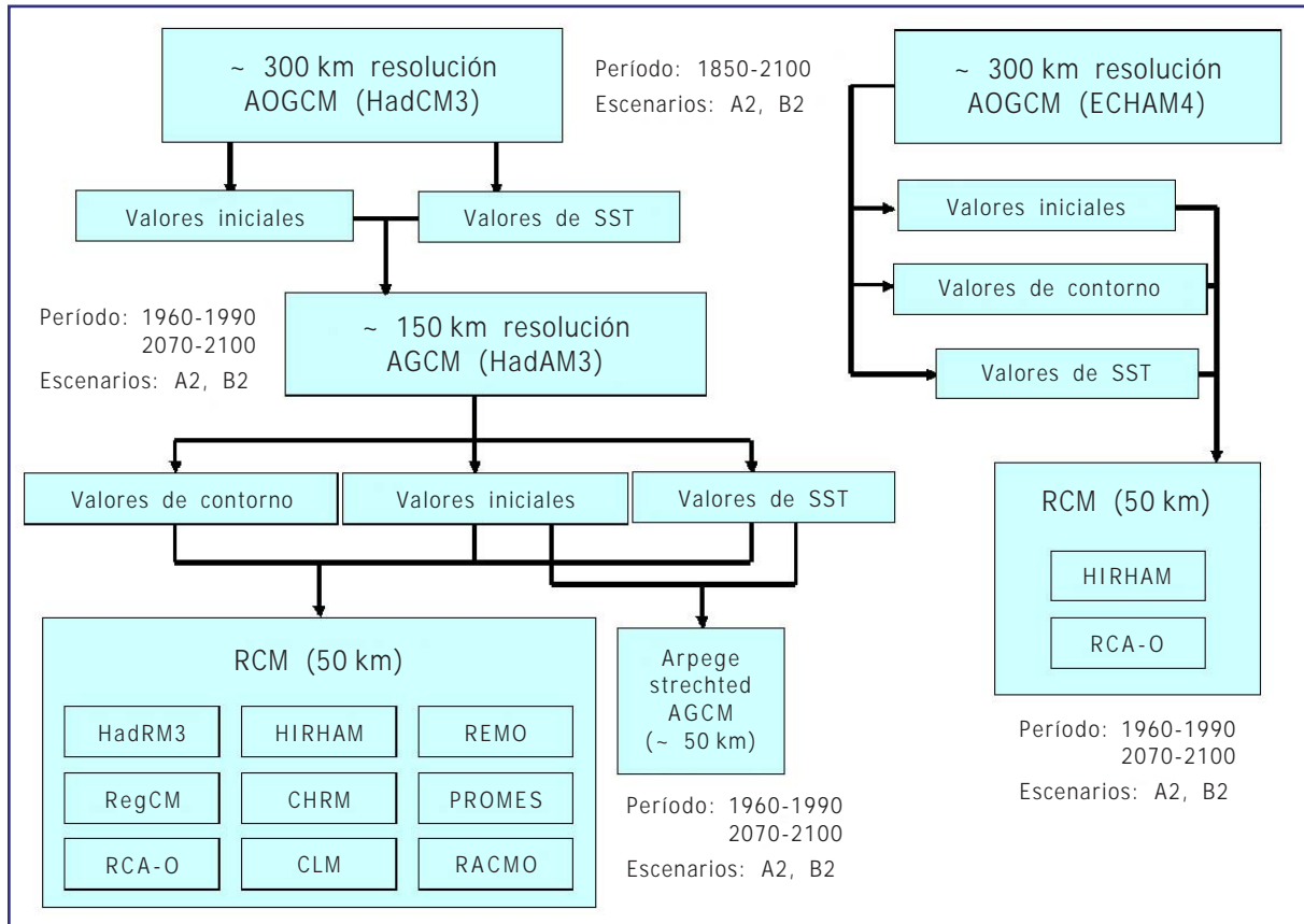
Figura 5.1. Esquema de las simulaciones realizadas en el proyecto PRUDENCE.
