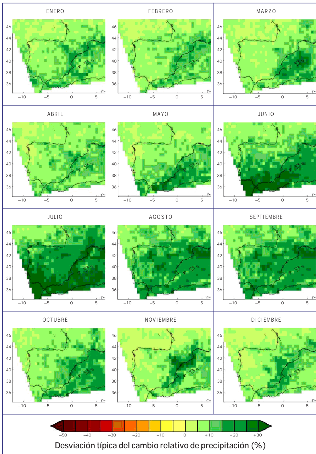
Figura 6.24. Distribución mensual de la desviación típica del cambio proyectado en la precipitación (%) para los diez modelos regionales de PRUDENCE en el período 2071-2100 respecto al clima actual (1961-1990) y para el escenario de emisión SRES A2.
