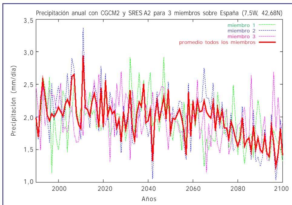
Figura 3.1. Evolución de la precipitación anual sobre un punto de rejilla (7,5°W, 42,68°N) en la Península Ibérica calculado para tres miembros de un ensemble del modelo global CGCM2 correspondientes al escenario de emisión SRES A2. La línea gruesa representa el promedio sobre todos los miembros del ensemble .
