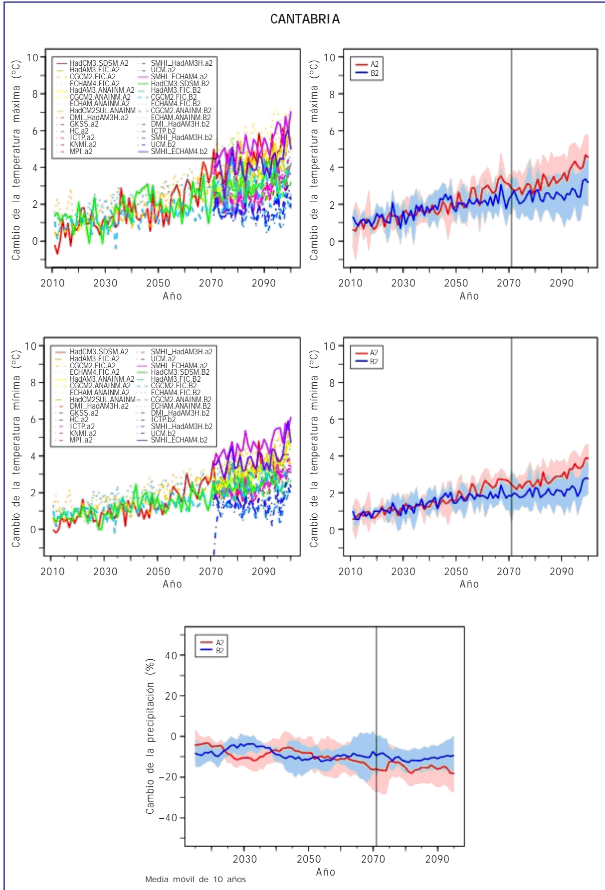
Figura B6. Igual que Figura B1, pero para Cantabria.
