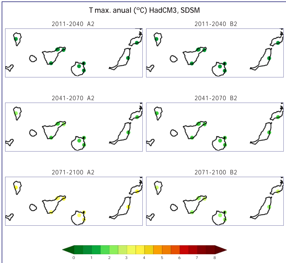
Figura 6.12. Cambio medio anual de temperatura máxima proyectada por el modelo global HadCM3 para los períodos 2011-2040 (arriba), 2041-2070 (centro) y 2071-2100 (abajo) respecto al clima actual (1961-1990) y regionalizado con el método de regresión (SDSM) para los escenarios de emisión SRES A2 (izda.) y B2 (dcha.).
