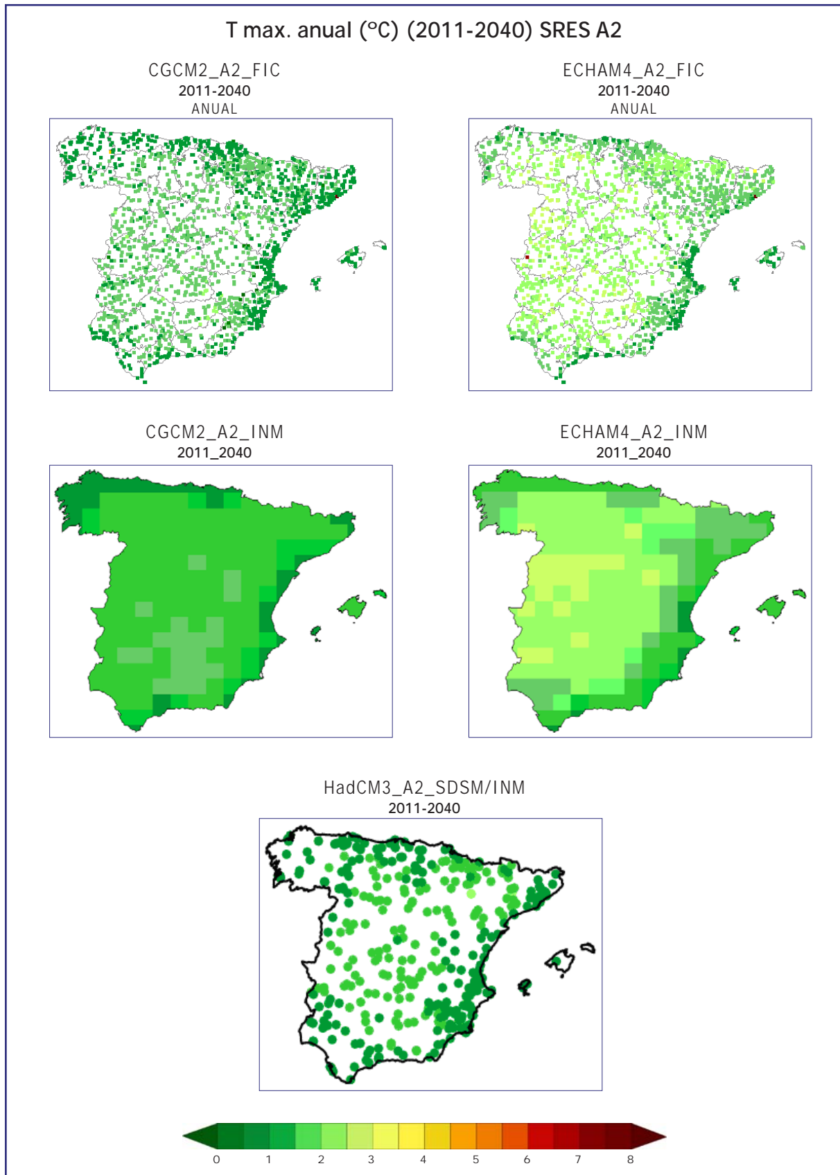
Figura 6.1. Comparación del cambio de temperatura máxima media anual para el período 2011-2040 respecto al período de control (1961-90) proporcionado por las proyecciones regionalizadas utilizando diferentes modelos globales (CGCM2 (izda.), ECHAM4-OPYC (der.), HadCM3 (centro abajo)) y diferentes técnicas de regionalización estadísticas (Anal_FIC(arriba), Anal_INM (centro), SDSM (abajo)). El escenario de emisión SRES común a todos los modelos es el A2.
