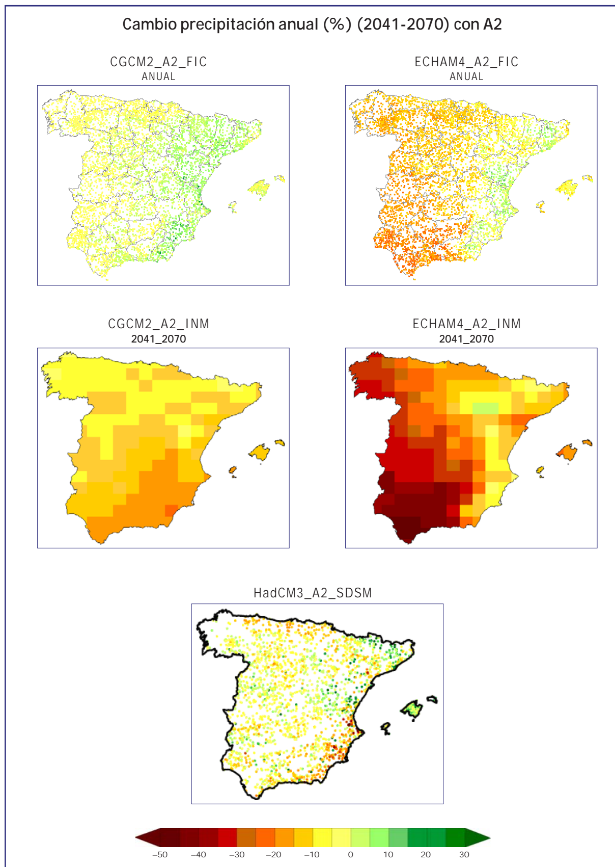
Figura 6.18. Comparación del cambio de precipitación anual para el período 2041-2070 respecto al período de control (1961-90) proporcionado por proyecciones regionalizadas utilizando diferentes modelos globales (HadCM3, CGCM2, ECHAM4-OPYC) y diferentes técnicas de regionalización estadísticas (Anal_FIC, Anal_INM, SDSM). El escenario de emisión SRES común a todos los modelos es el A2.
