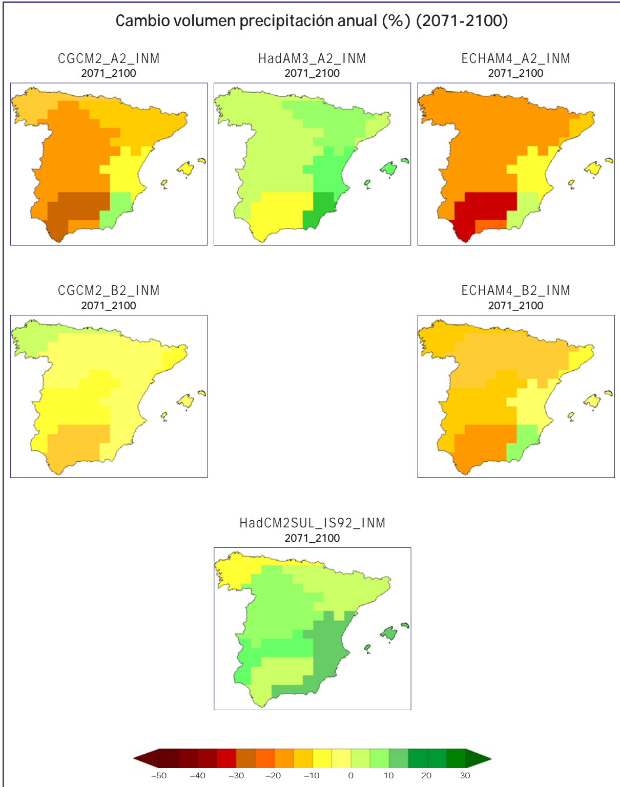
Figura 6.33. Comparación del cambio del volumen de precipitación anual por cuencas hidrográficas para el período 2071-2100 respecto al período de control (1961-90) proporcionado por proyecciones regionalizadas utilizando diferentes modelos globales (HadCM2SUL, HadAM3H, CGCM2, ECHAM4-OPYC) y las técnicas de regionalización de los índices de circulación. La primera fila corresponde al escenario de emisión SRES A2, la segunda fila al escenario SRES B2 y la tercera fila al escenario IS92a.
