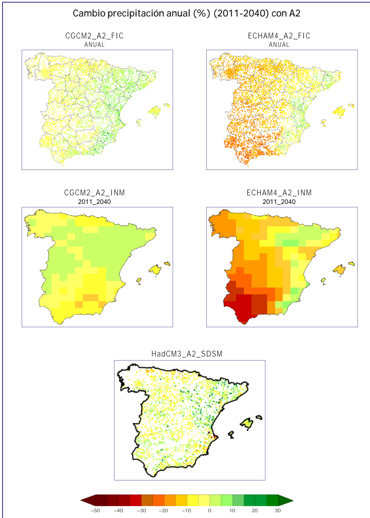
Figura 6.17. Comparación del cambio de precipitación anual para el período 2011-2040 respecto al período de control (1961-90) proporcionado por proyecciones regionalizadas utilizando diferentes modelos globales (HadCM3, CGCM2, ECHAM4-OPYC) y diferentes técnicas de regionalización estadísticas (Anal_FIC, Anal_INM, SDSM). El escenario de emisión SRES común a todos los modelos es el A2.
