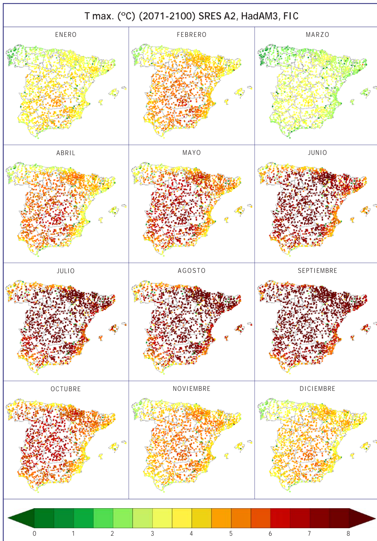
Figura 6.4. Cambio medio mensual de temperatura máxima proyectado para el período 2071-2100 respecto al clima actual (1961-1990) por el modelo global HadAM3H y regionalizado con el método de análogos (FIC) para el escenario de emisión A2.
