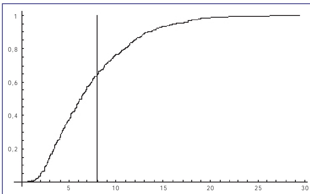
Figura 2.3. Función de distribución del estadístico del test SNHT. La probabilidad acumulada se muestra en ordenadas, el estadístico en abscisas y la línea vertical marca el valor crítico del estadístico.
