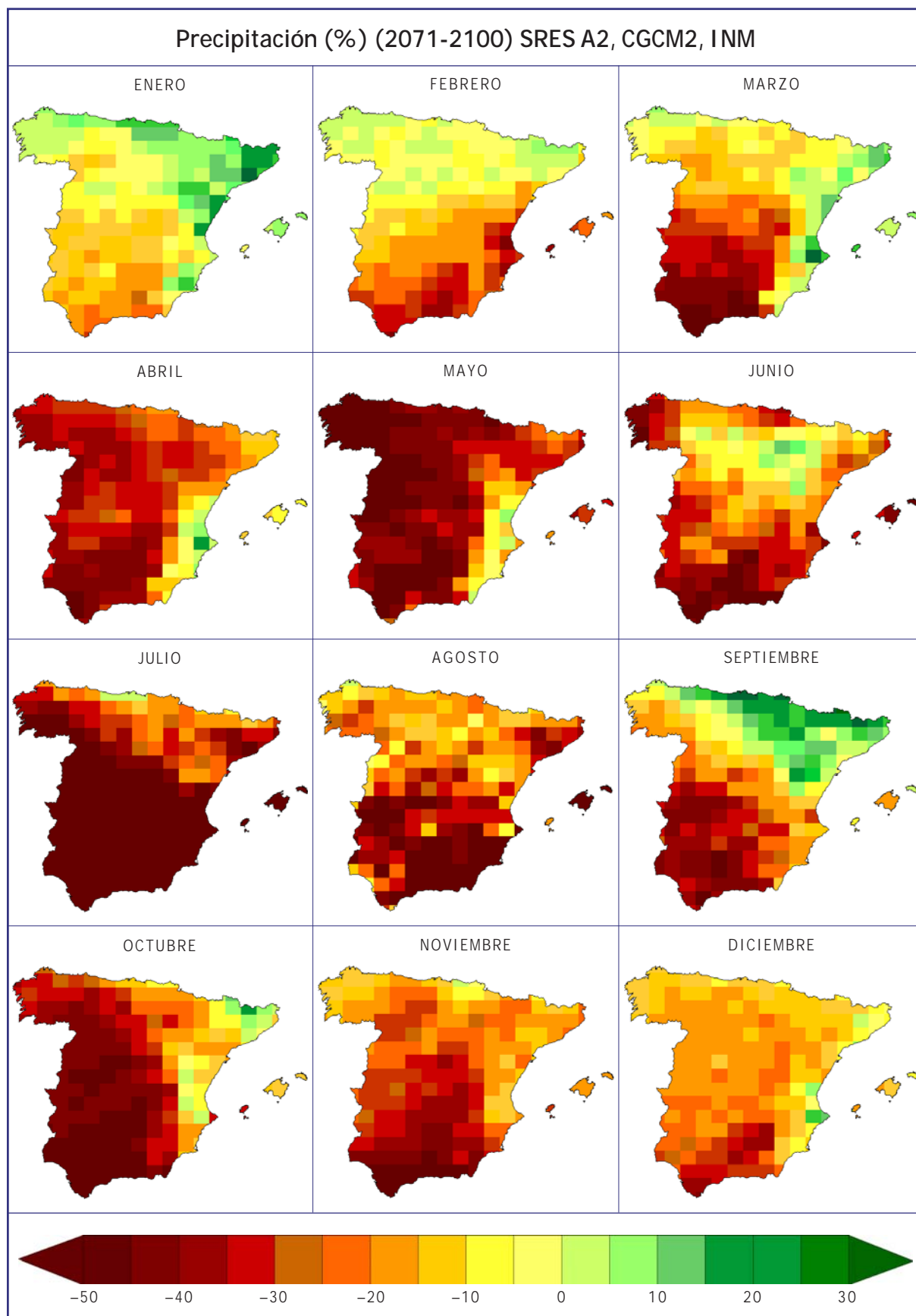
Figura 6.20. Cambio medio mensual de precipitación (%) proyectado para el periodo 2071-2100 respecto al clima actual (1961-1990) por el modelo global CGCM2 y regionalizado con el método de análogos (INM) para el escenario de emisión A2.
