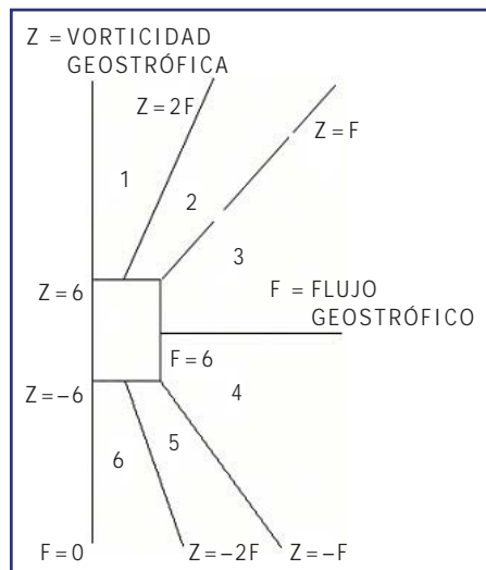
Figura 5.6. Asignación del valor diario del índice ciclónico según sean los valores del flujo y vorticidad geostrófica. En las zonas 1 y 6 se asigna valor +2 y -2, respectivamente; en las zonas 2 y 5 se asigna el valor +1 y -1, respectivamente; en las zonas 3 y 4 se asigna el valor 0. En la zona 7, de valores pequeños, también se asigna el valor 0.
