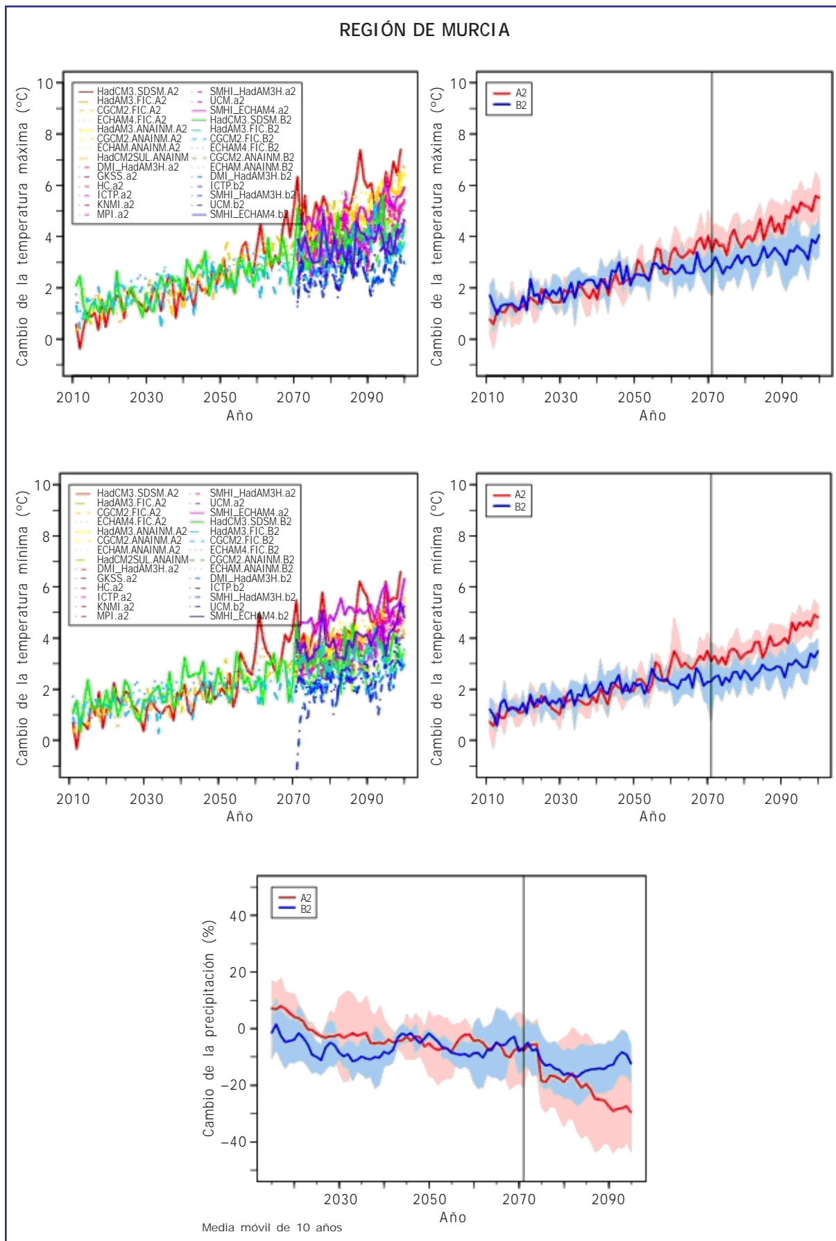
Figura B14. Igual que Figura B1, pero para la Región de Murcia.
