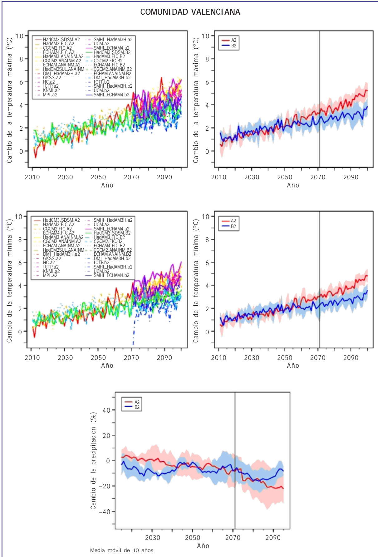
Figura B17. Igual que Figura B1, pero para la Comunidad Valenciana.
