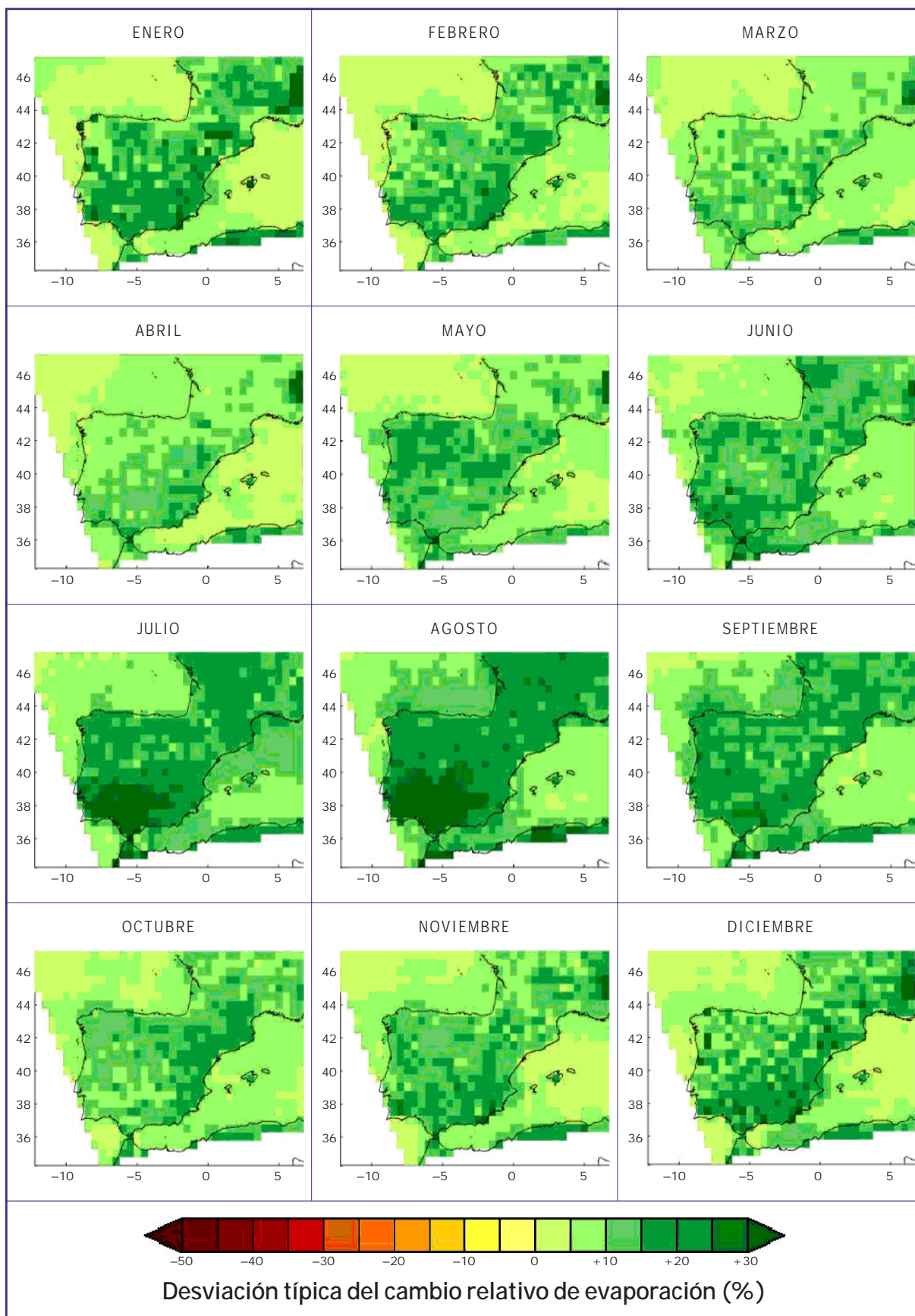
Figura 6.30. Distribución mensual de la desviación típica del cambio proyectado en la precipitación (%) para los diez modelos regionales de PRUDENCE en el período 2071-2100 respecto al clima actual (1961-1990) y para el escenario de emisión SRES A2.
