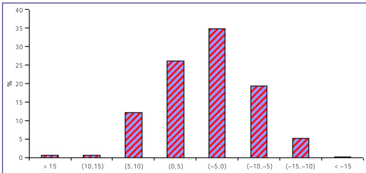
Figura 2.6. Histograma de las pendientes (en °C/100 años) de las diferencias con la serie de referencia para las series de temperatura inhomogéneas al 5% con el test de Mann.
