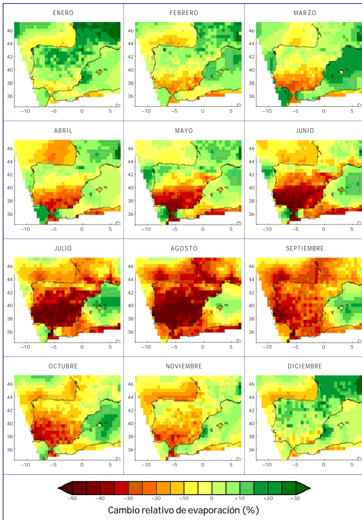
Figura 6.29. Cambio medio mensual de evapotranspiración (%) proyectado para el periodo 2071-2100 respecto al clima actual (1961-1990) por el modelo global HadAM3H y regionalizado con el promedio de los RCM de PRUDENCE para el escenario de emisión A2.
