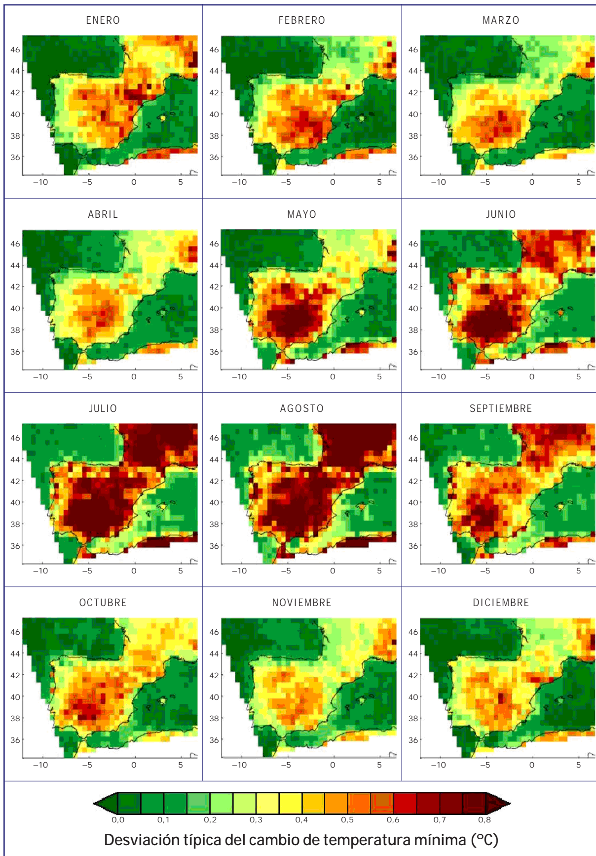
Figura 6.16. Distribución mensual de la desviación típica del cambio proyectado en la temperatura mínima para los diez modelos regionales de PRUDENCE en el período 2071-2100 respecto al clima actual (1961-1990) y para el escenario de emisión SRES A2.
