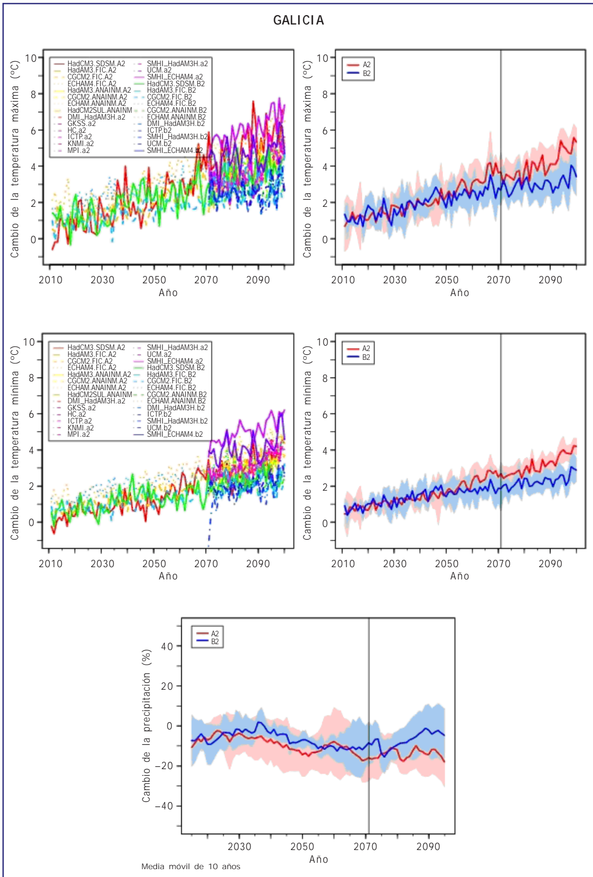
Figura B11. Igual que Figura B1, pero para Galicia.
