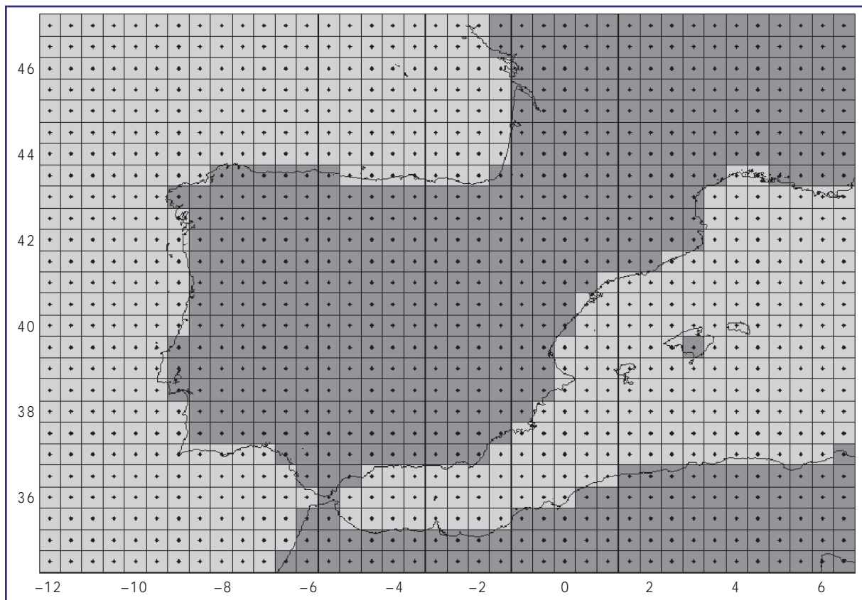
Figura A2. Dominio y malla comunes donde se han interpolado los resultados de todos los RCM de PRUDENCE. Las celdillas sombreadas corresponden a tierra y las blancas a mar.
