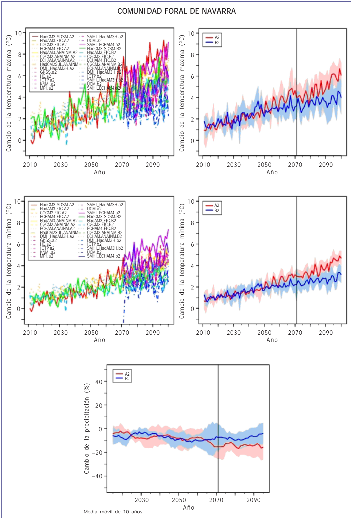
Figura B15. Igual que Figura B1, pero para la Comunidad Foral de Navarra.
