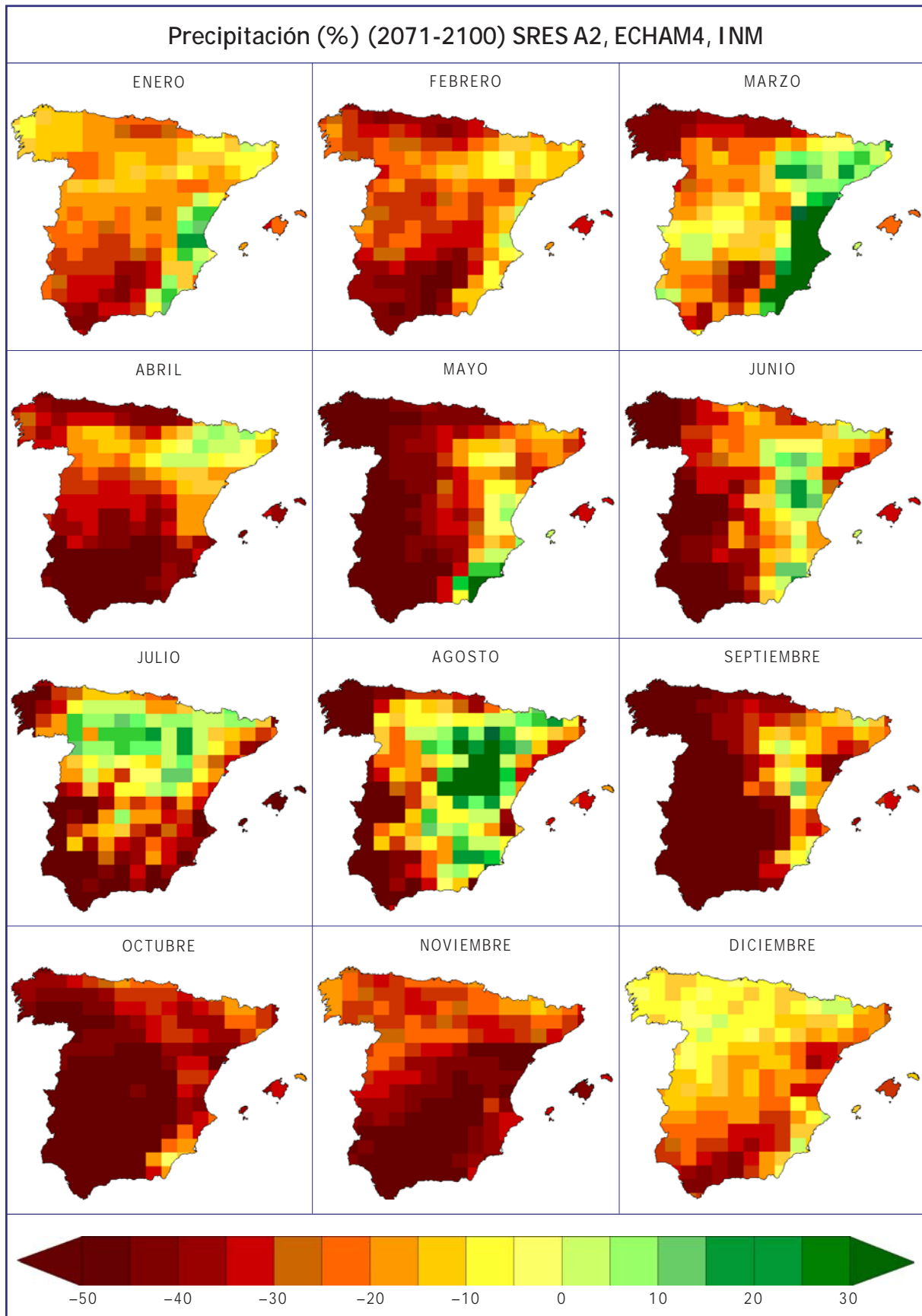
Figura 6.21. Cambio medio mensual de precipitación (%) proyectado para el periodo 2071-2100 respecto al clima actual (1961-1990) por el modelo global ECHAM4-OPYC y regionalizado con el método de análogos (INM) para el escenario de emisión A2.
