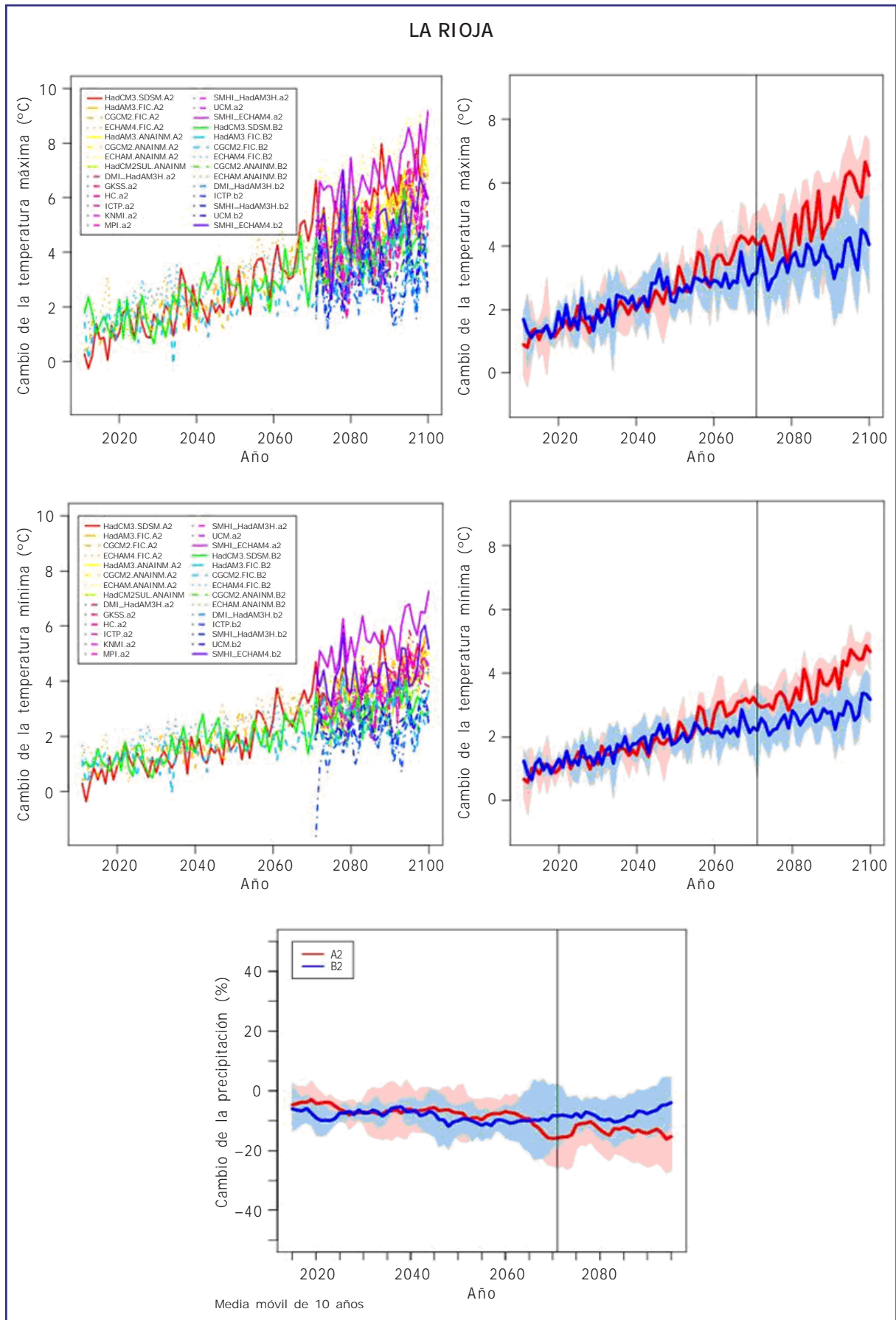
Figura B12. Igual que Figura B1, pero para La Rioja.
