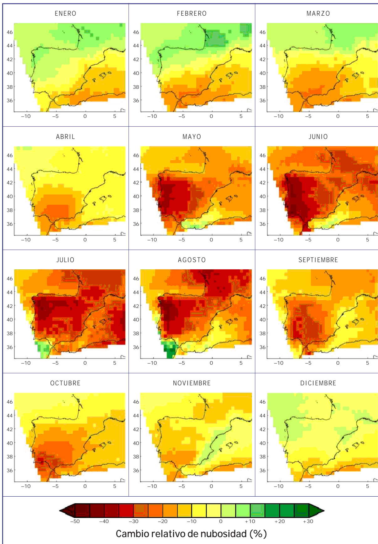
Figura 6.27. Cambio medio mensual de nubosidad (%) proyectado para el período 2071-2100 respecto al clima actual (1961-1990) por el modelo global HadAM3H y regionalizado con el promedio de los RCM de PRUDENCE para el escenario de emisión A2.
