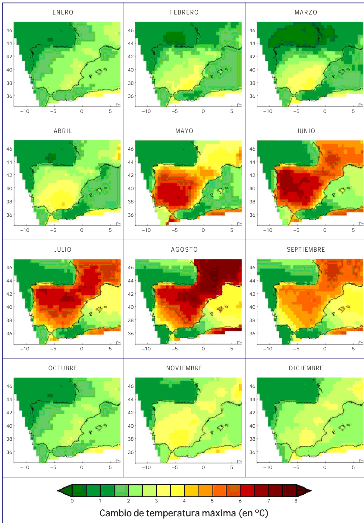
Figura 6.7. Cambio medio mensual de temperatura máxima proyectado para el período 2071-2100 respecto al clima actual (1961-1990) por el modelo global HadAM3H y regionalizado con el promedio de los RCM de PRUDENCE para el escenario de emisión A2.
