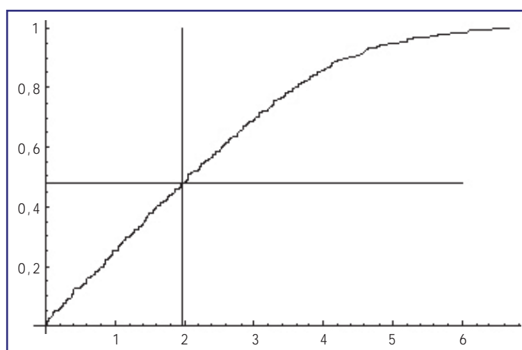
Figura 2.5. Función de distribución del estadístico estandarizado del test de Mann. La probabilidad acumulada se muestra en ordenadas, el estadístico en abscisas y la línea vertical marca el valor crítico del estadístico.
