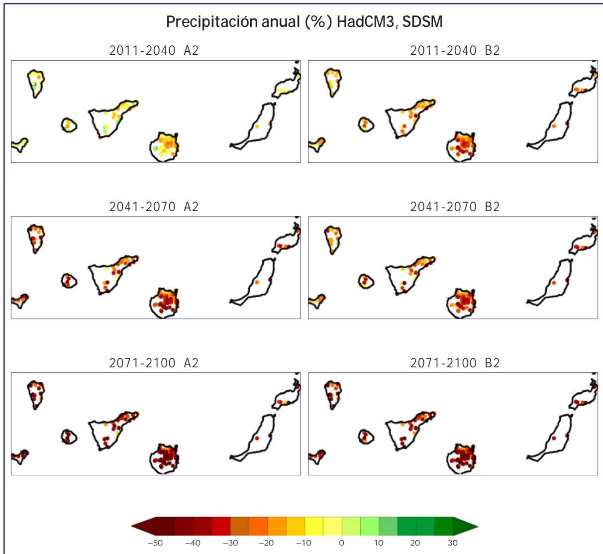
Figura 6.25. Cambio de precipitación anual proyectada por el modelo global HadCM3 para los periodos 2011-2040 (arriba), 2041-2070 (centro) y 2071-2100 (abajo) respecto al clima actual (1961-1990) y regionalizado con el método de regresión (SDSM) para los escenarios de emisión SRES A2 (izda.) y B2 (dcha.).
