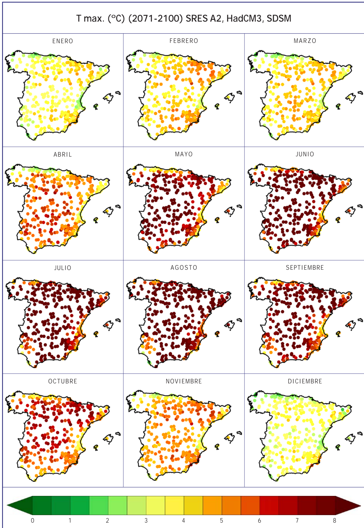
Figura 6.5. Cambio medio mensual de temperatura máxima proyectado para el período 2071-2100 respecto al clima actual (1961-1990) por el modelo global HadCM3 y regionalizado con el método SDSM para el escenario de emisión A2.
