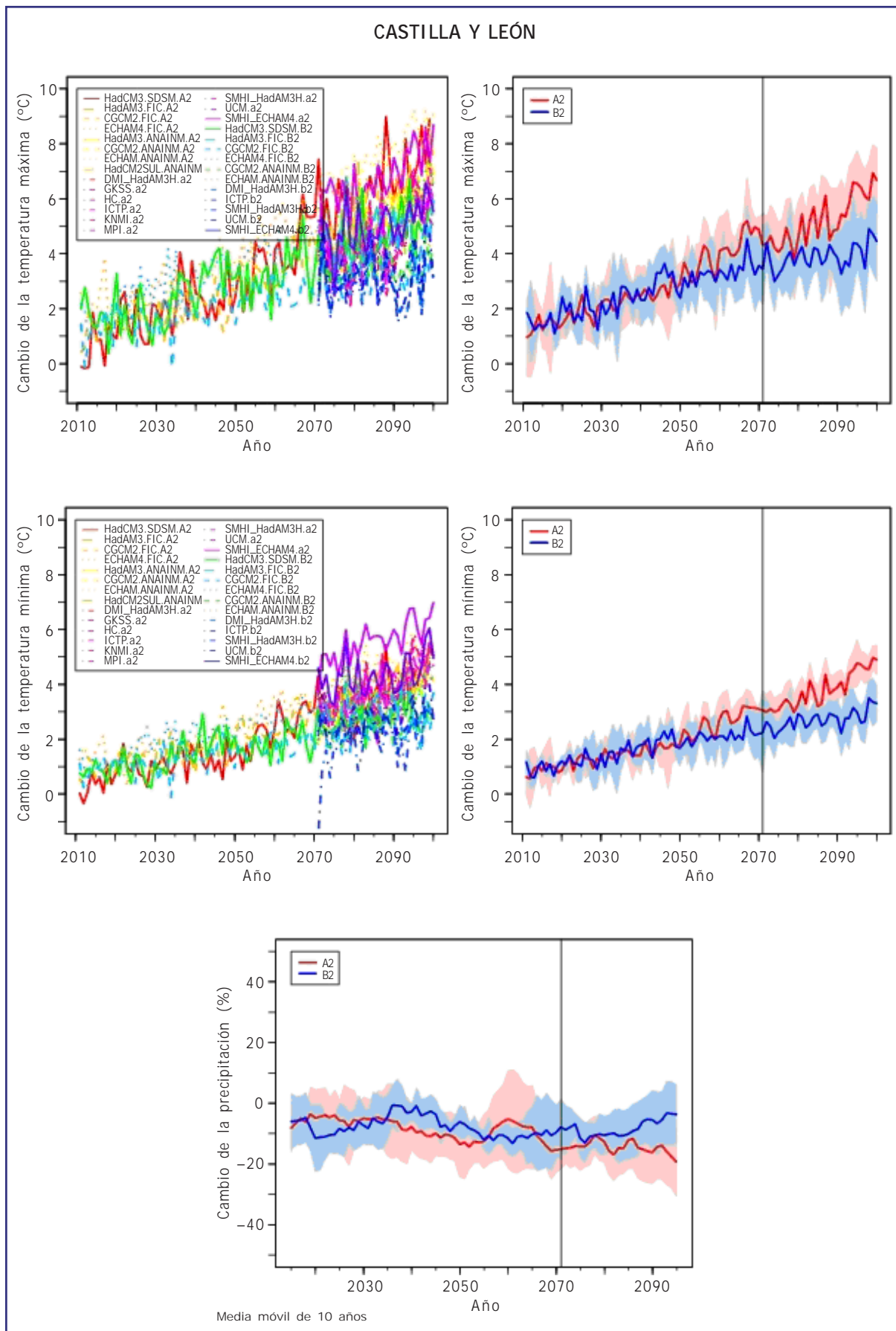
Figura B8. Igual que Figura B1, pero para Castilla y León.
